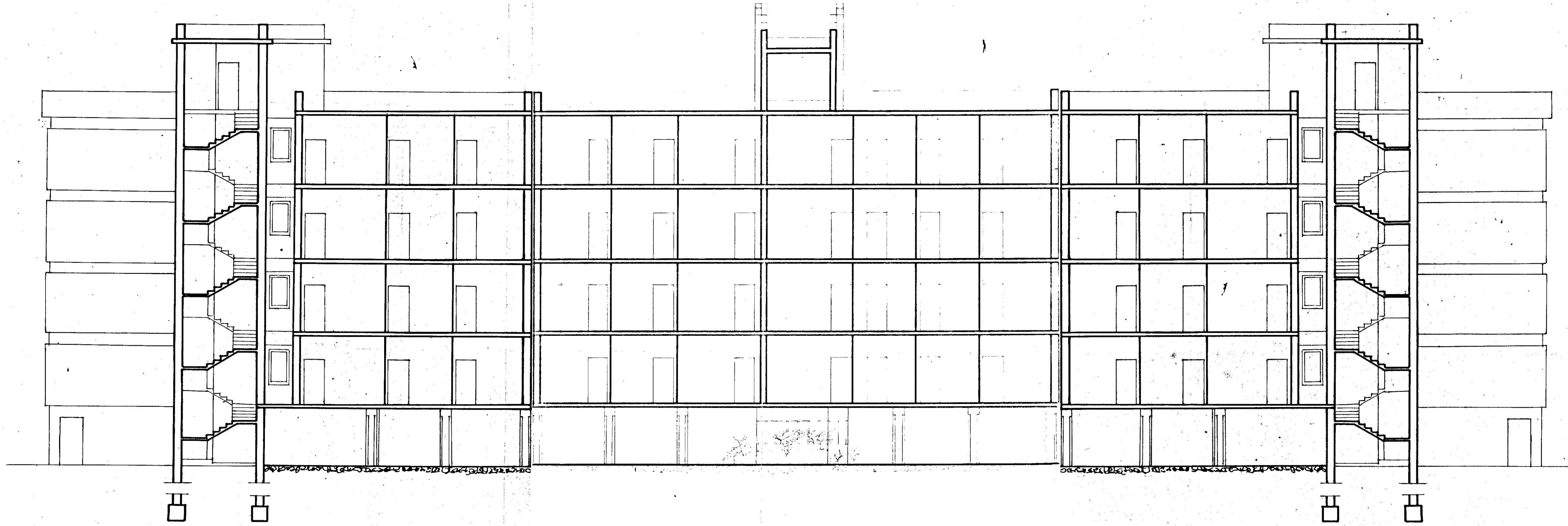
SEZIONE 'CC.'
