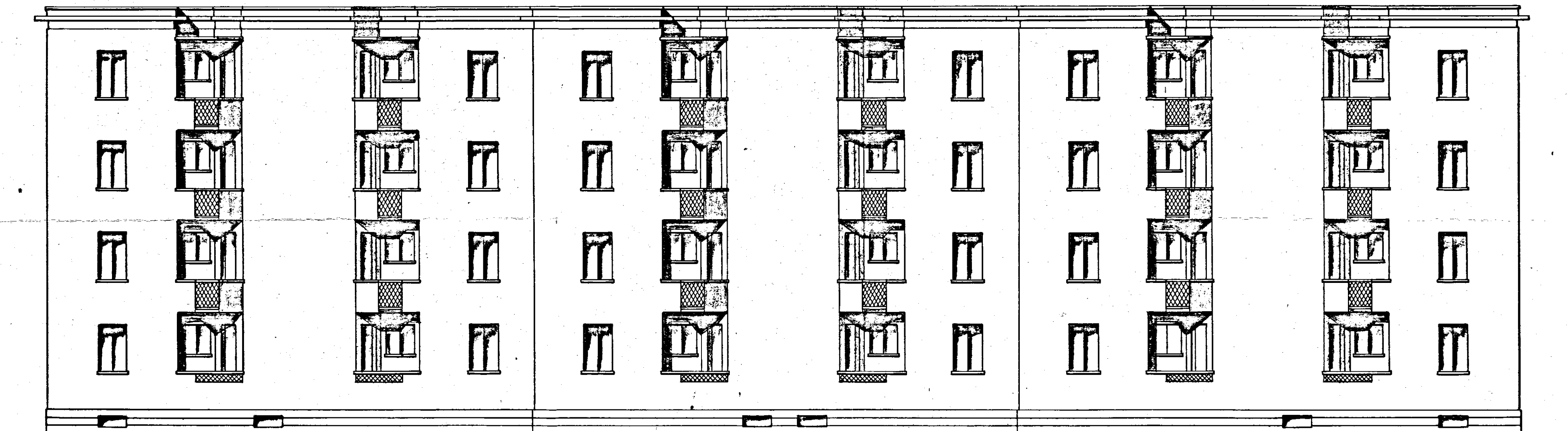
PROSPETTO POSTERIORE
