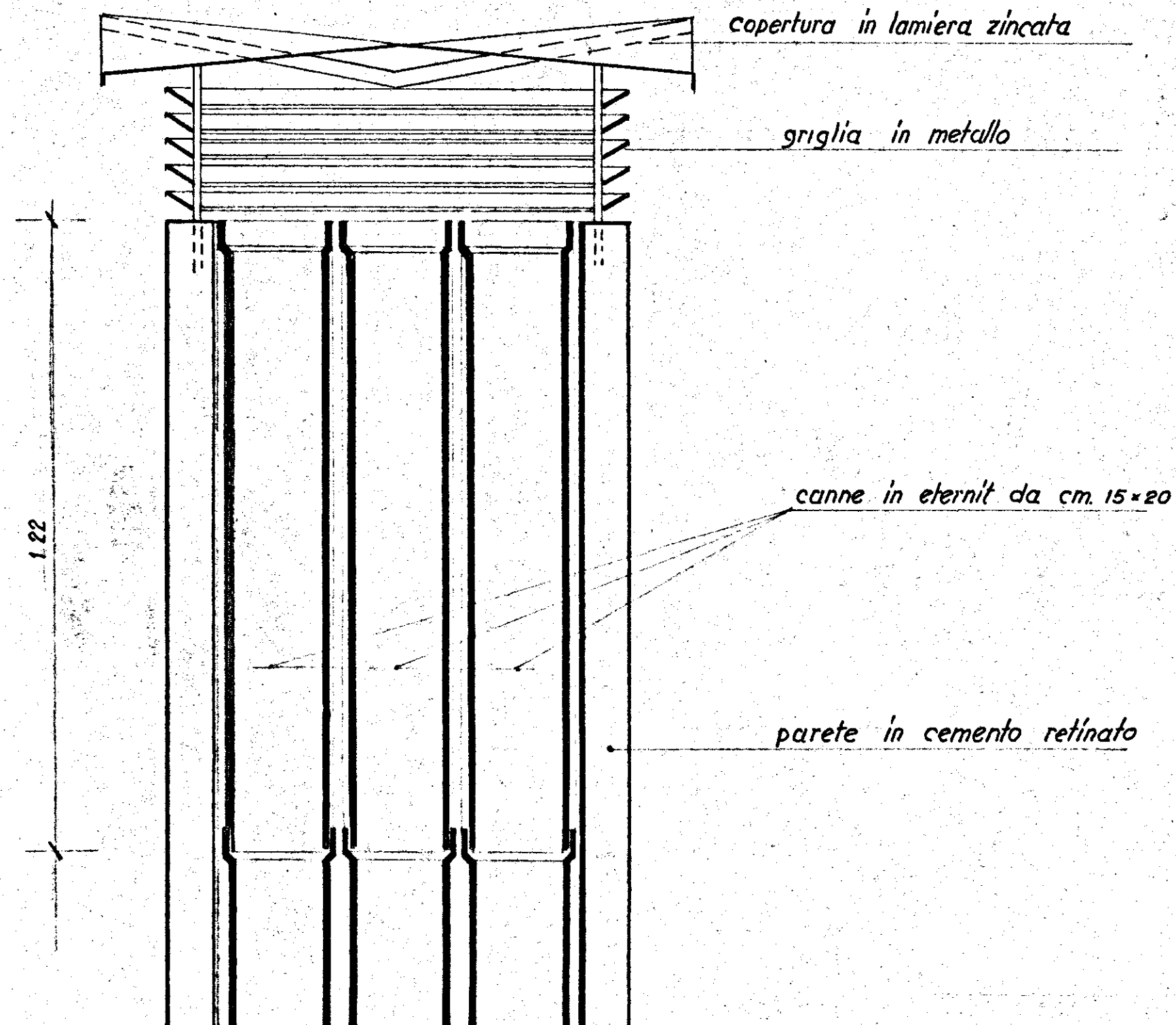
SEZIONE A-B
