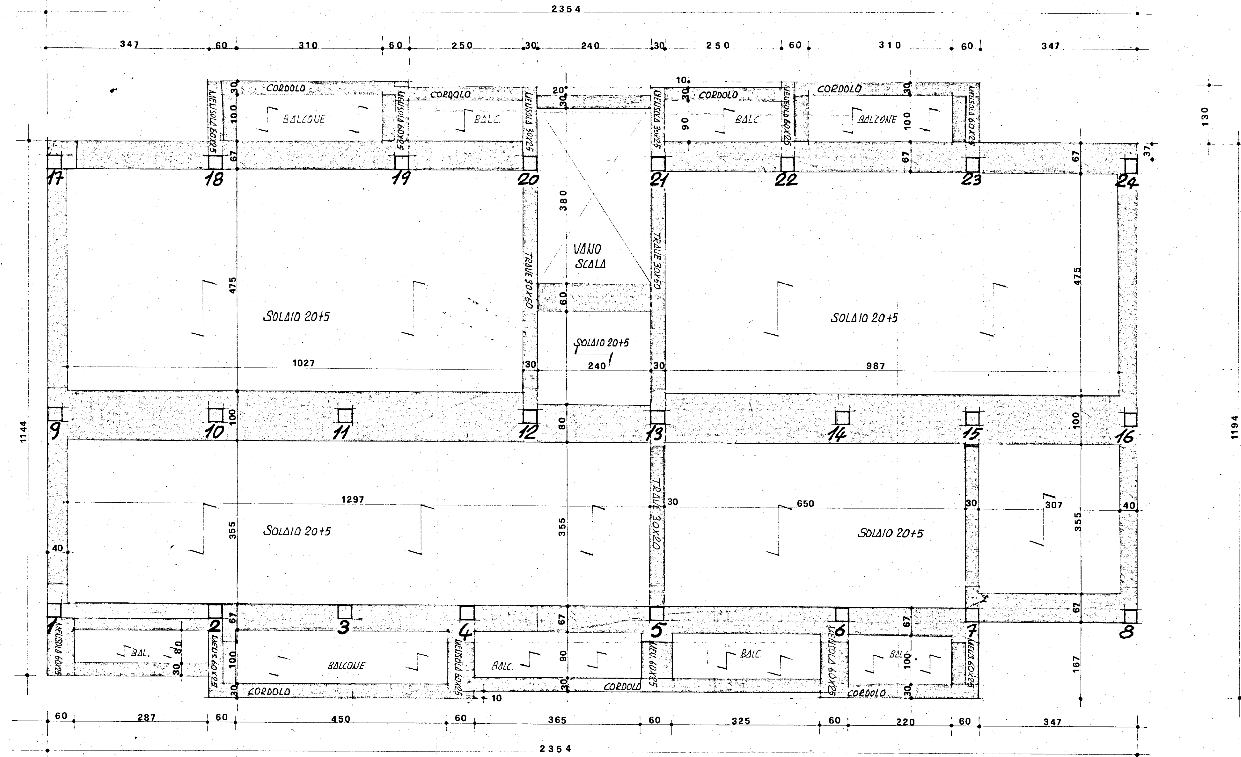
PIANTA COPERTURA PIANO TIPO
