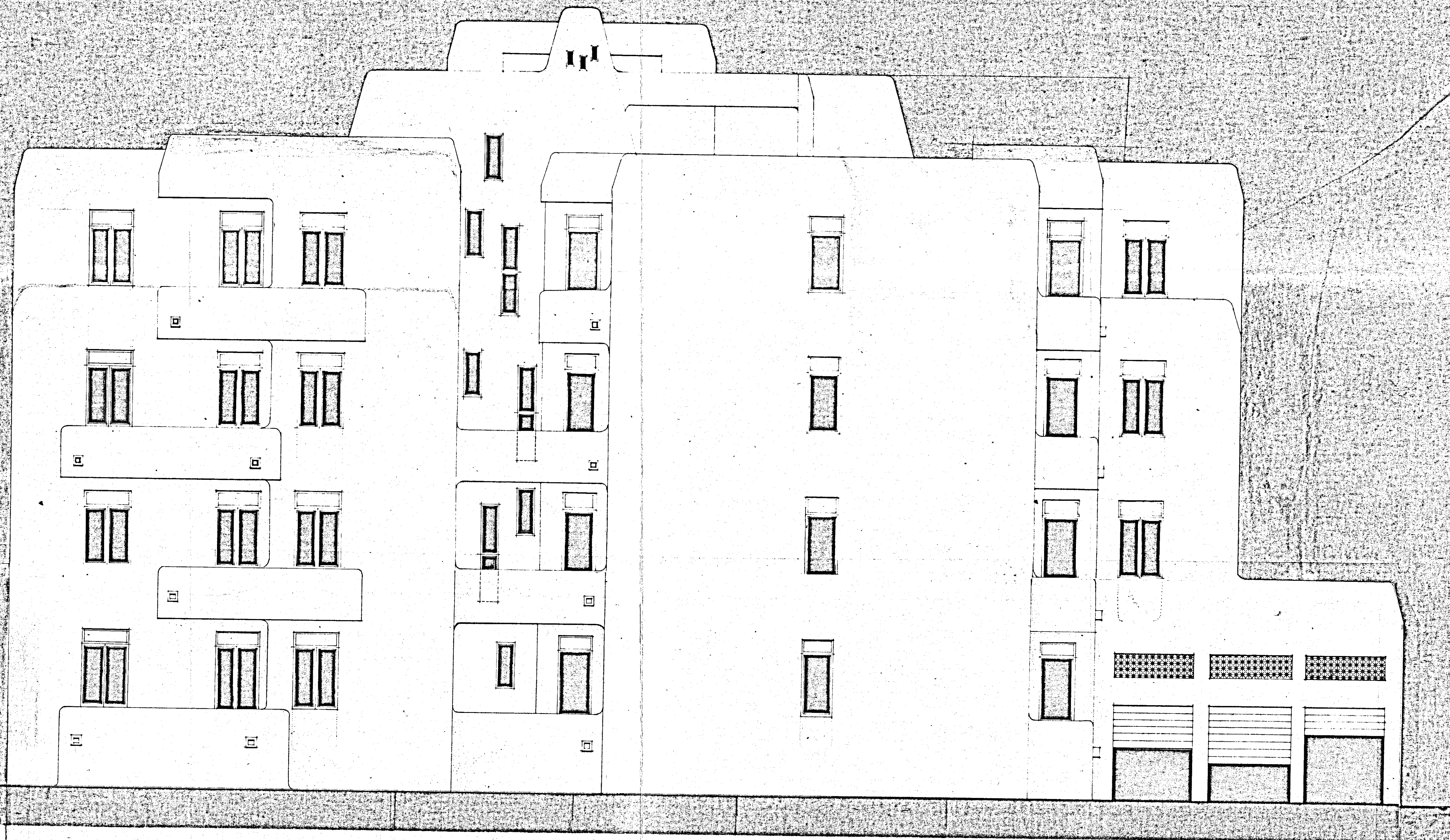
PROSPETTO -D-
