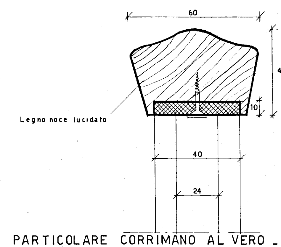
PARTICOLARE CORRIMANO AL VERO .
