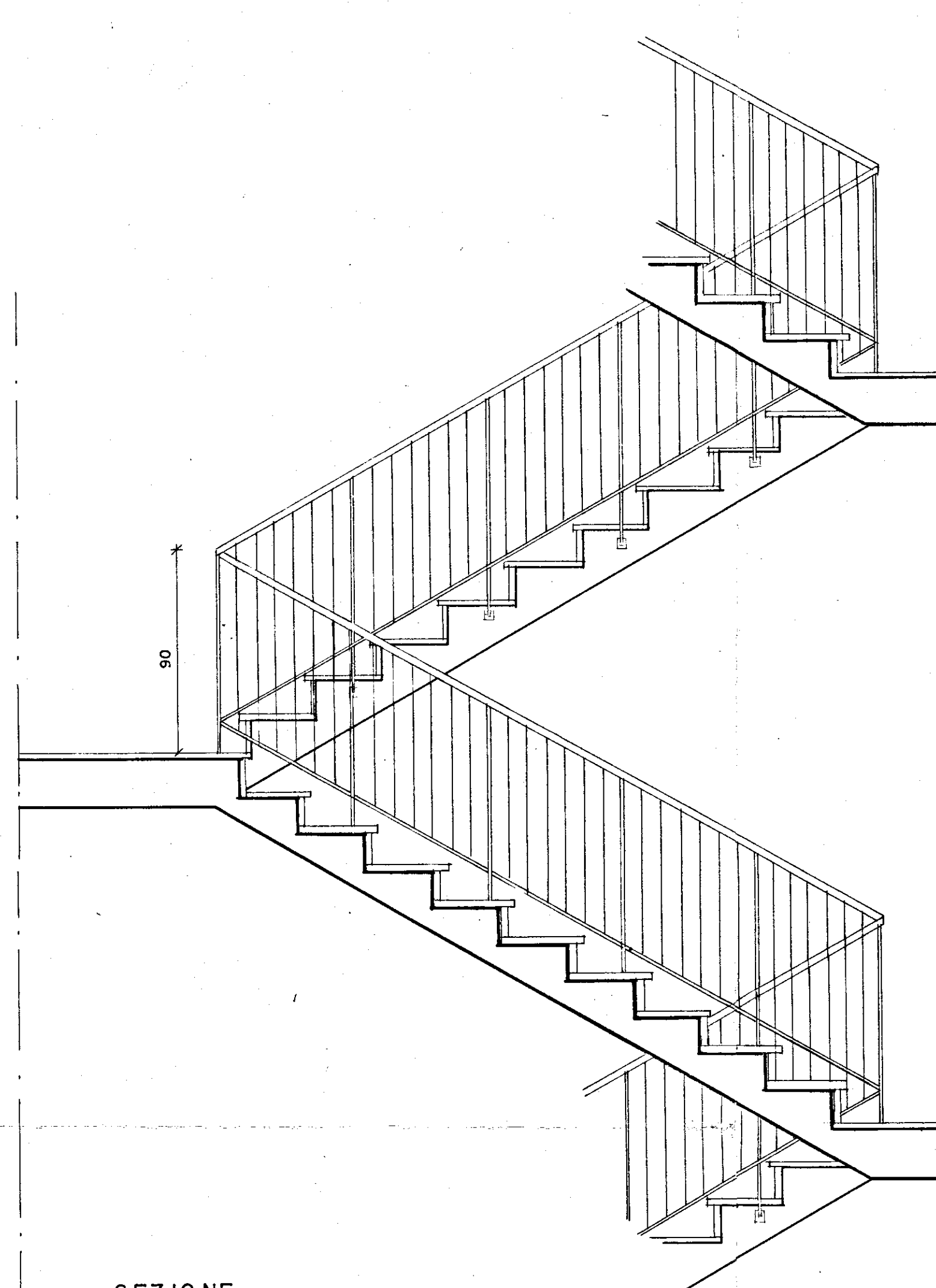
- SEZIONE -
