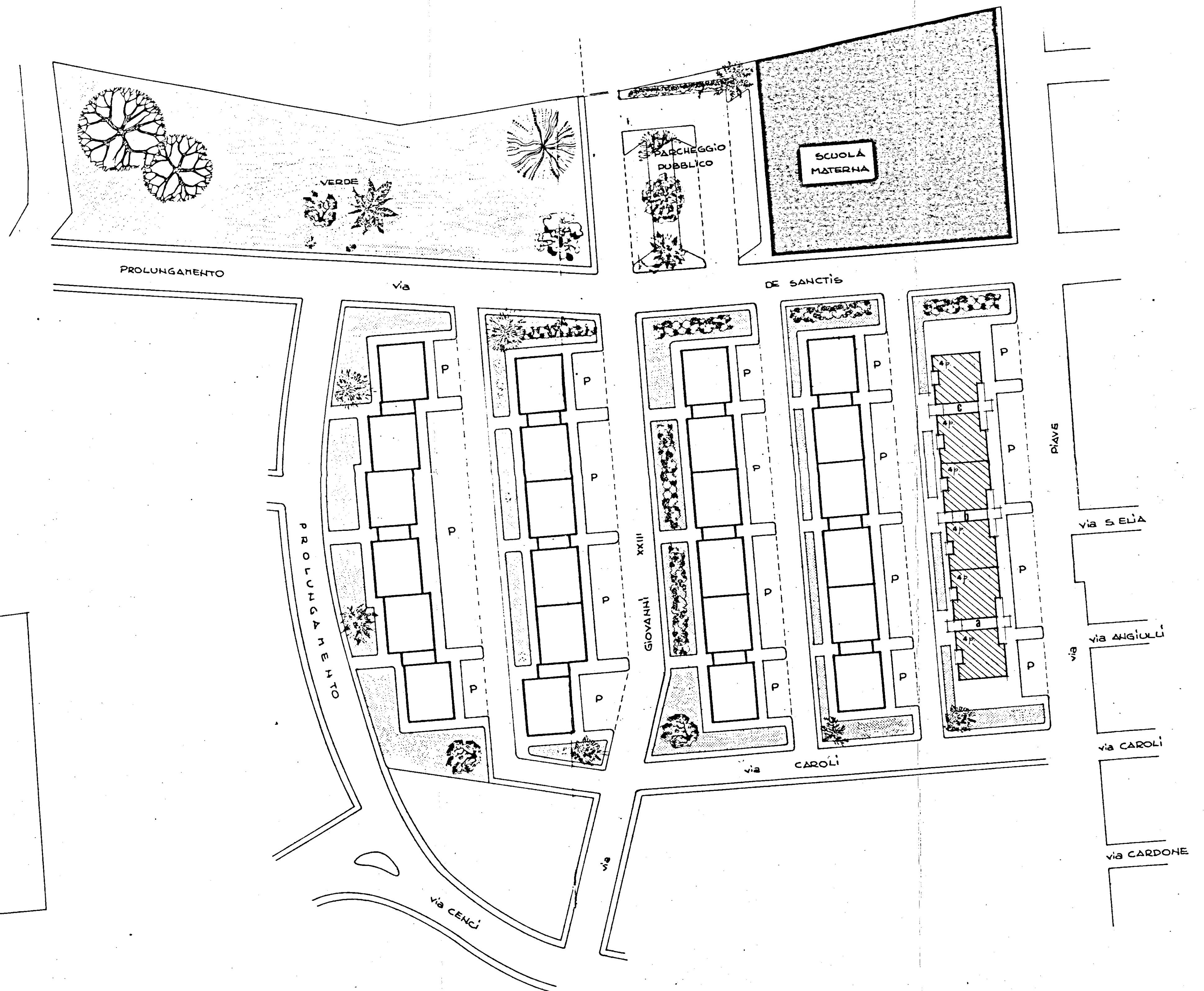
SCHEMA DI SISTEMAZIONE SPAZI ESTERNI E DEI FRONTI DEGLI EDIFICI SCALA 1:500
