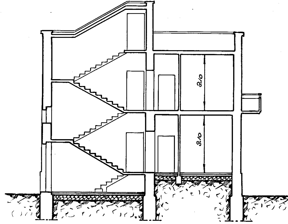
Sezione A-B
