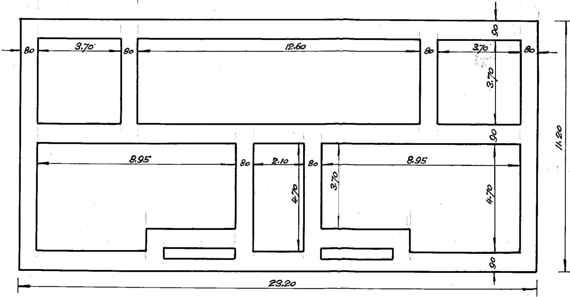
Fondazioni
