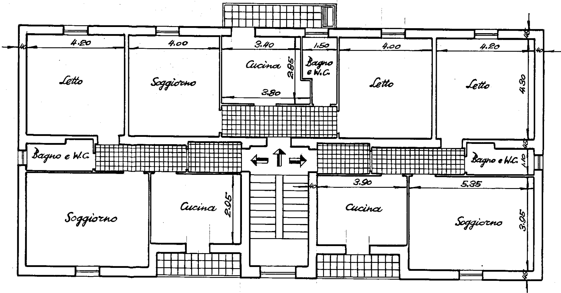
Primo piano
