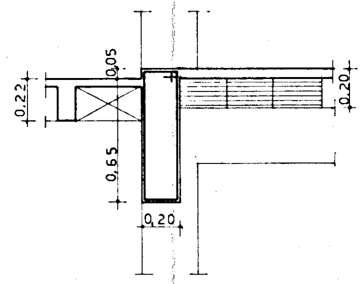
Particolare trave 5-10,5-10 in corrispondenza del pianerottolo di arrivo: rapp. 1:20
