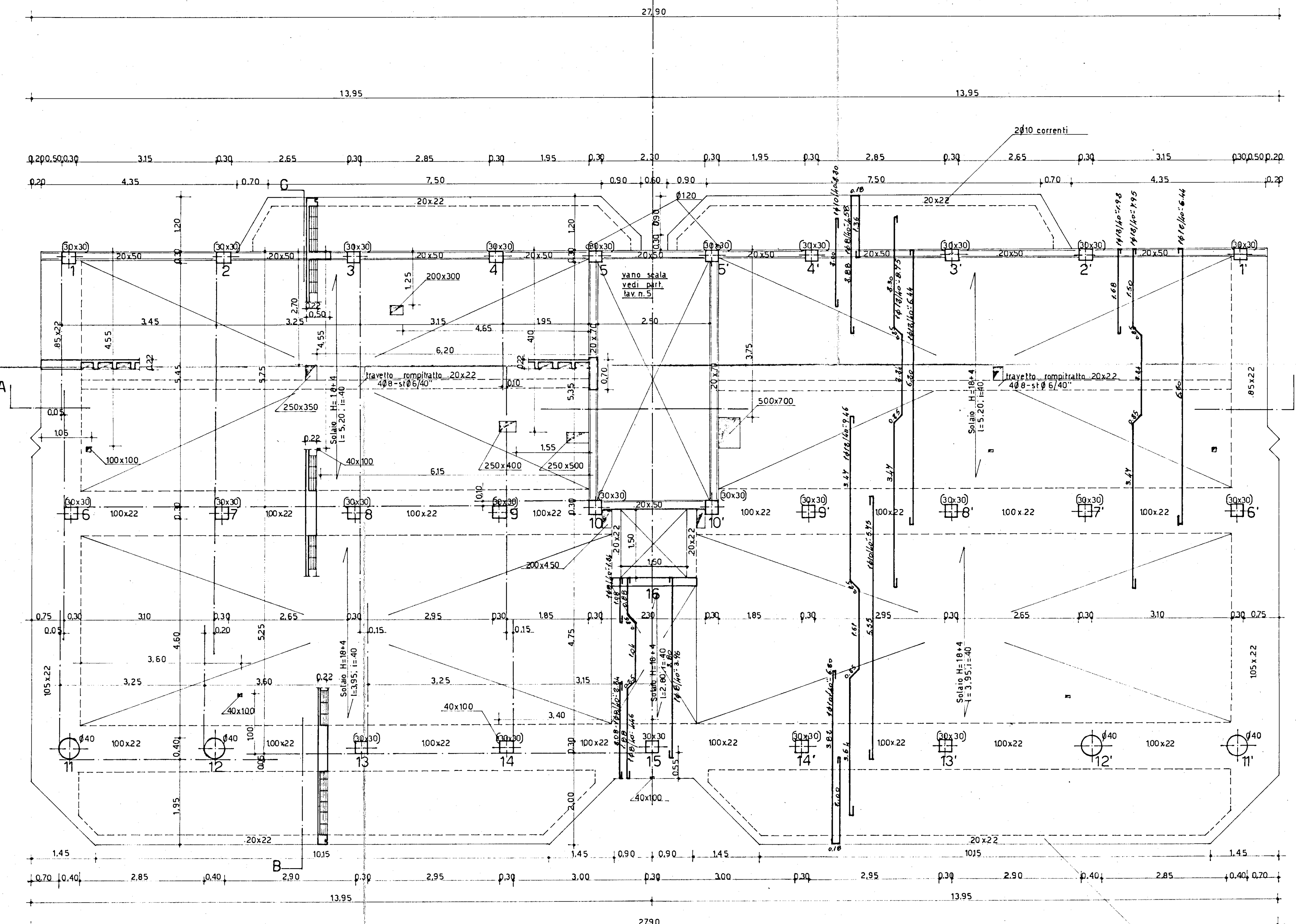
SEZIONE A-B
