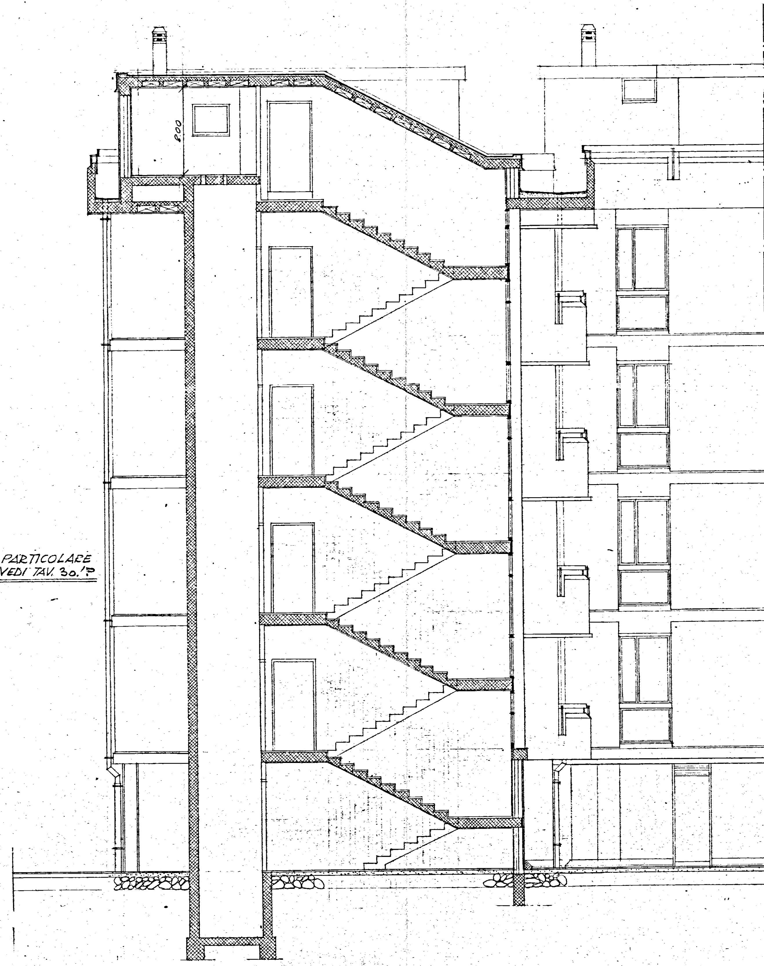
SEZIONE X-Y
