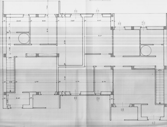
primo piano
