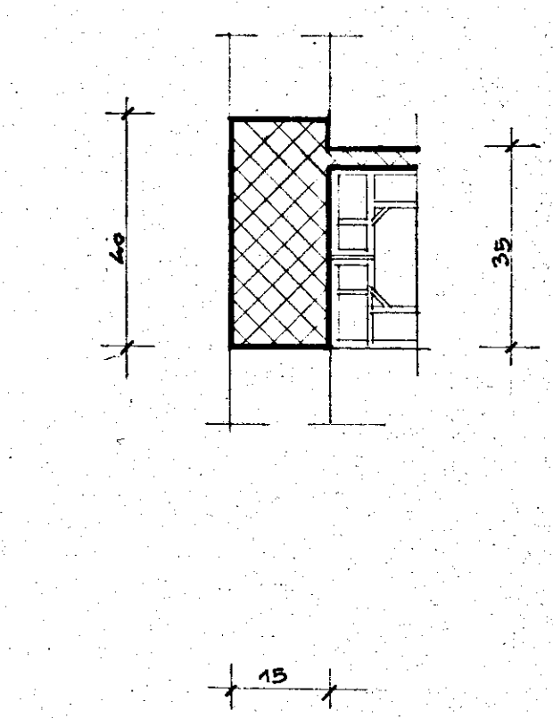
SEZIONE E-F
