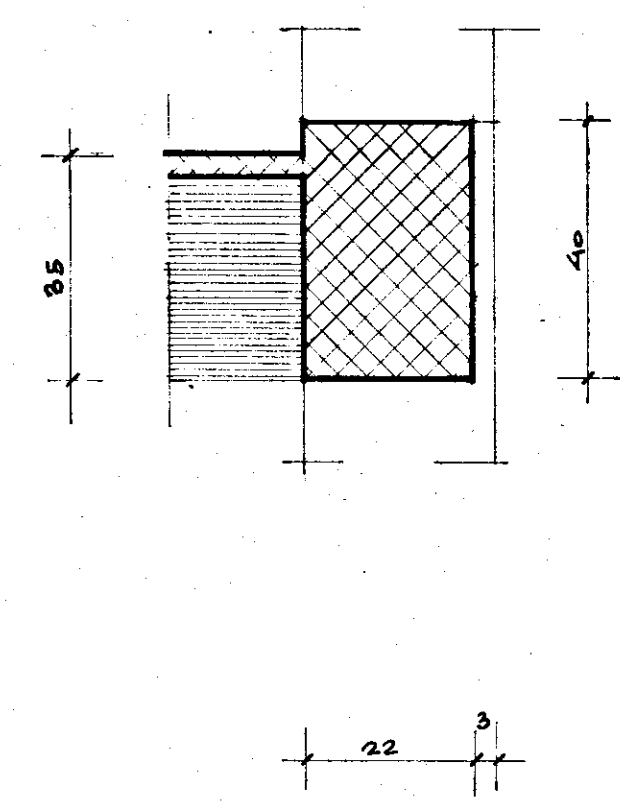
SEZIONE A-B
