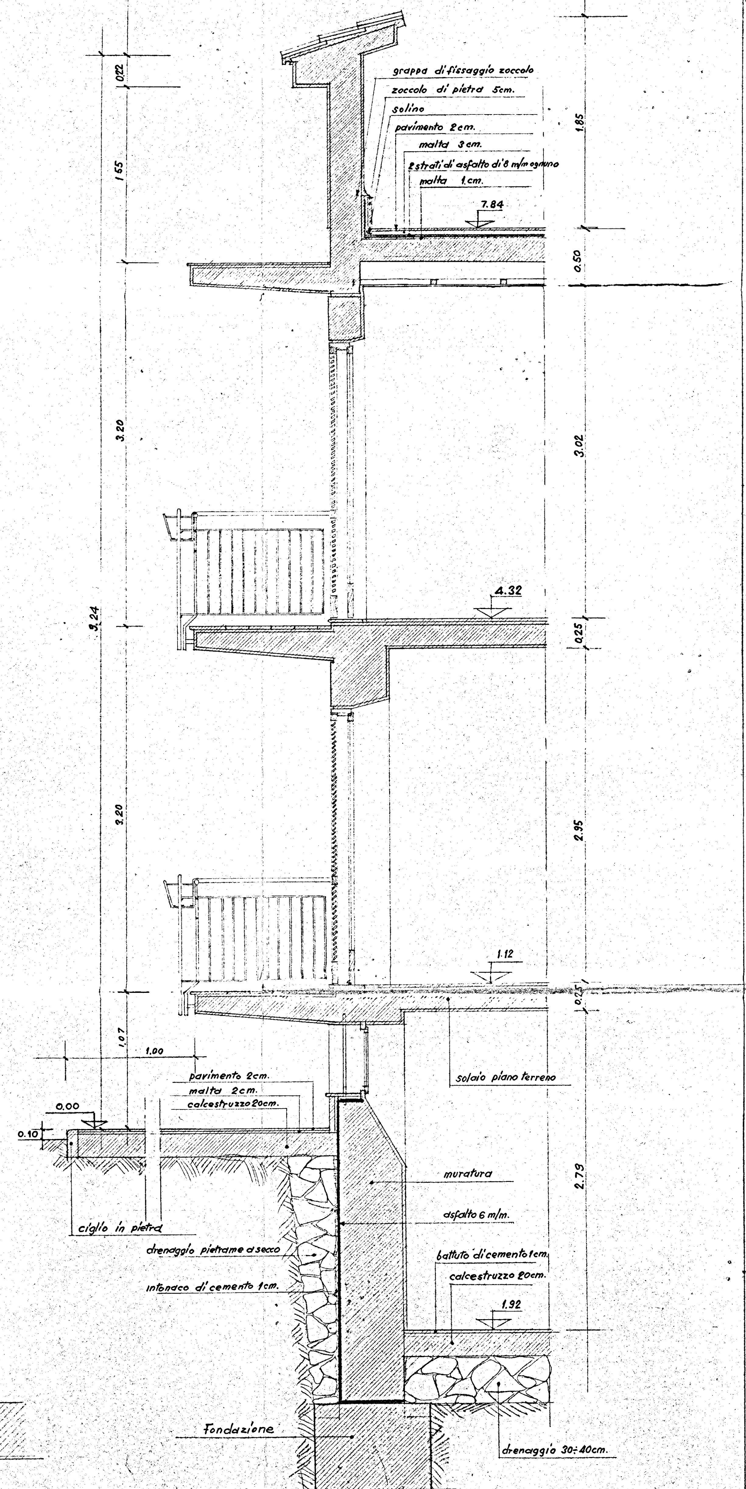
SEZIONE A-A
