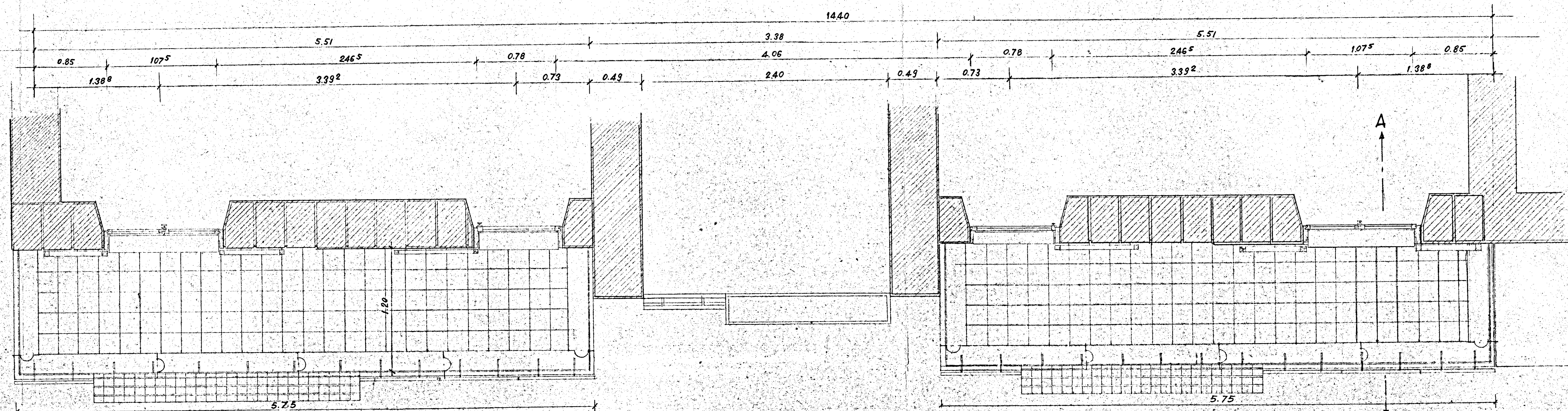
PIANTA
