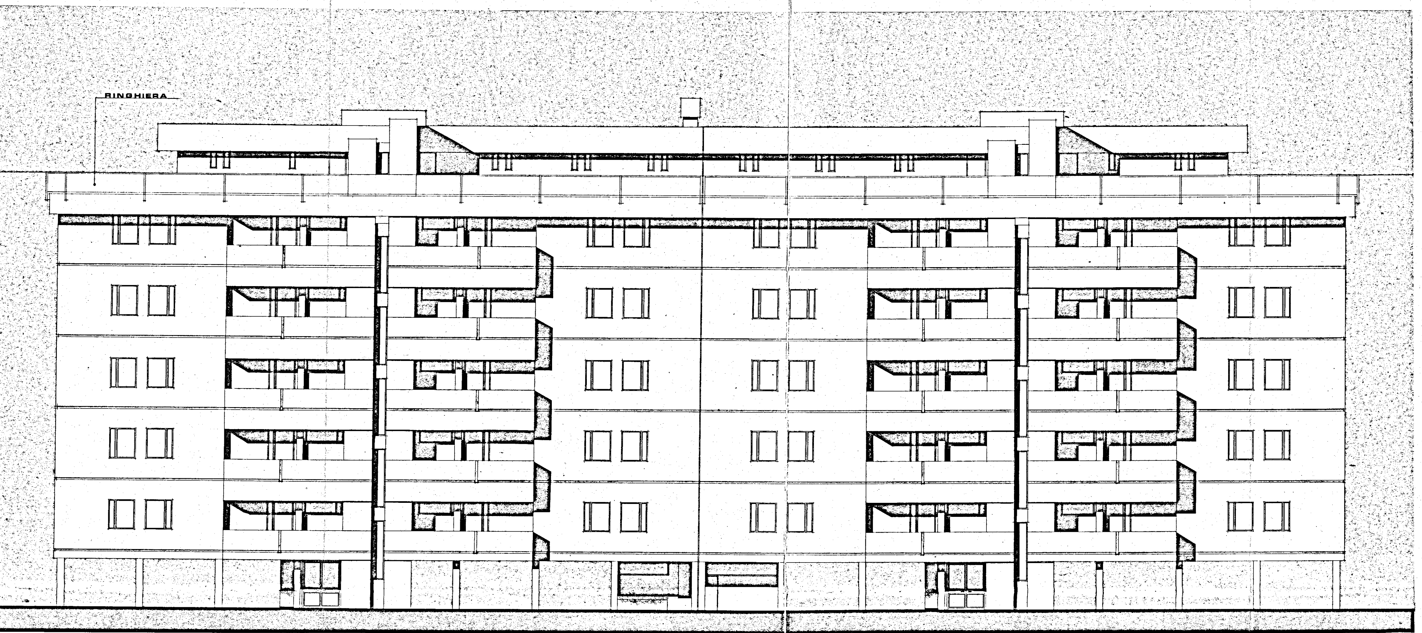
PROSPETTO OVEST
