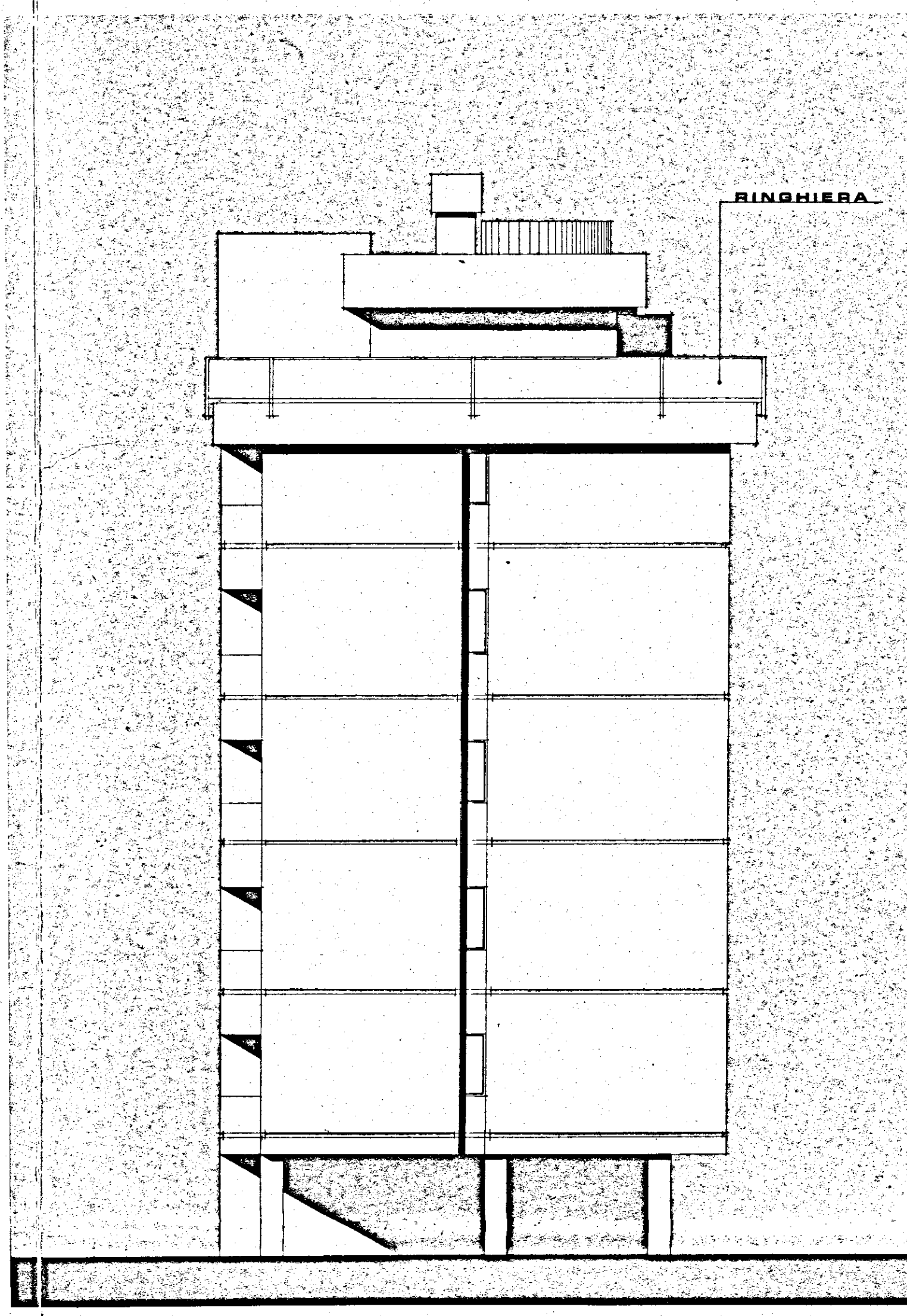
PROSPETTO SUD
