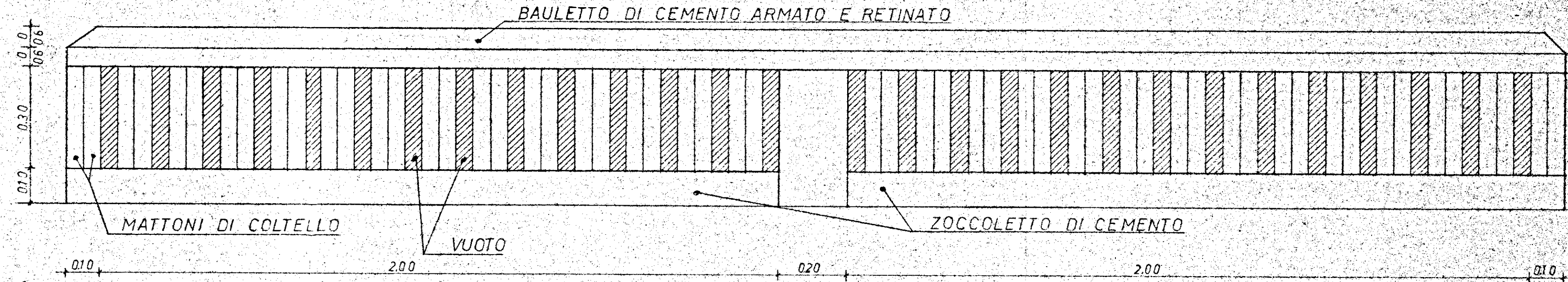
PARTICOLARE DELL'AERATORE
