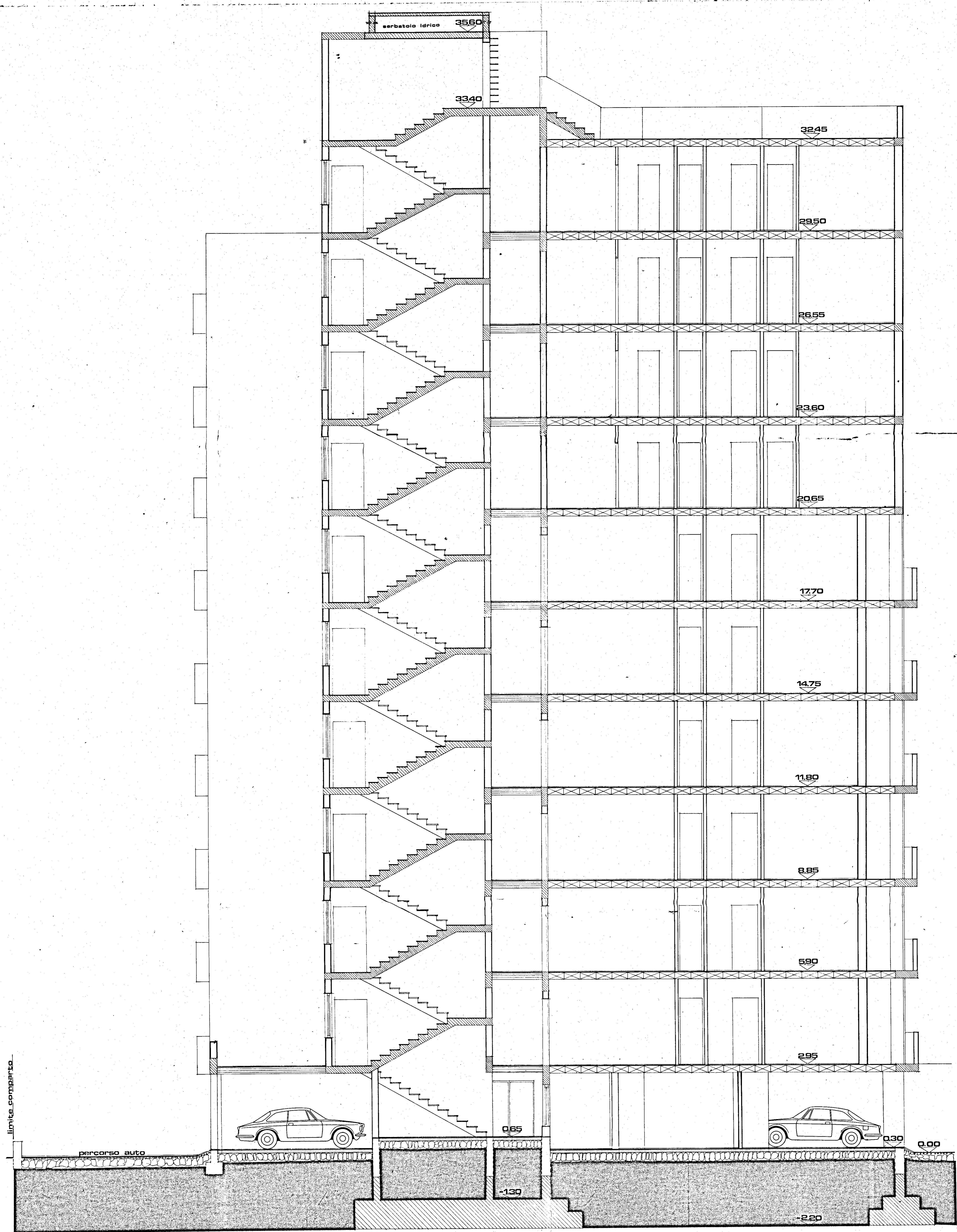
SEZIONE B-B
