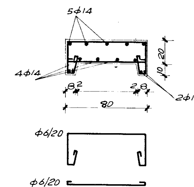
SEZIONE TRAVE DI CORONAMENTO PORTICO RAPPR. 1:20
