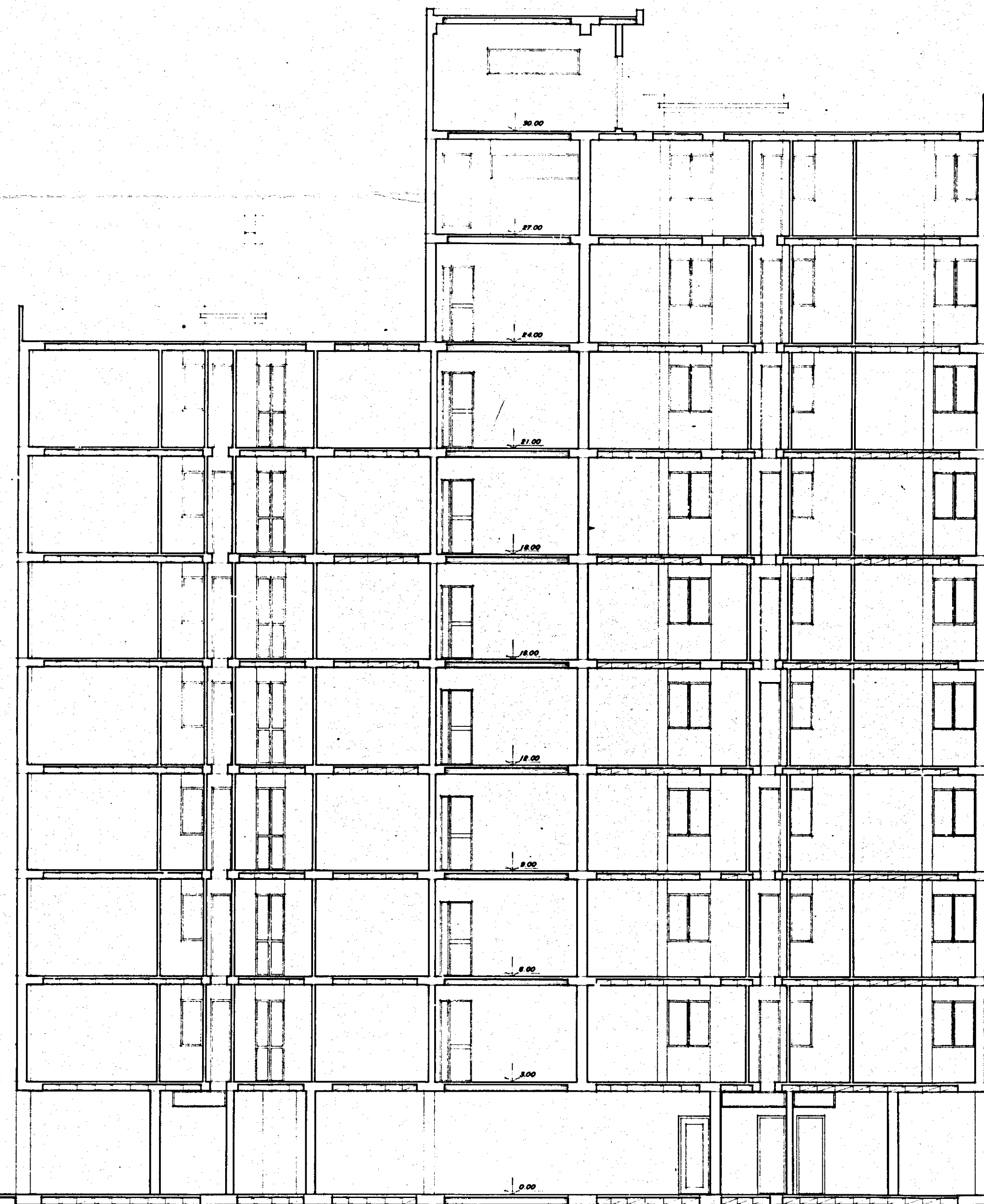
SEZIONE Y-Y
