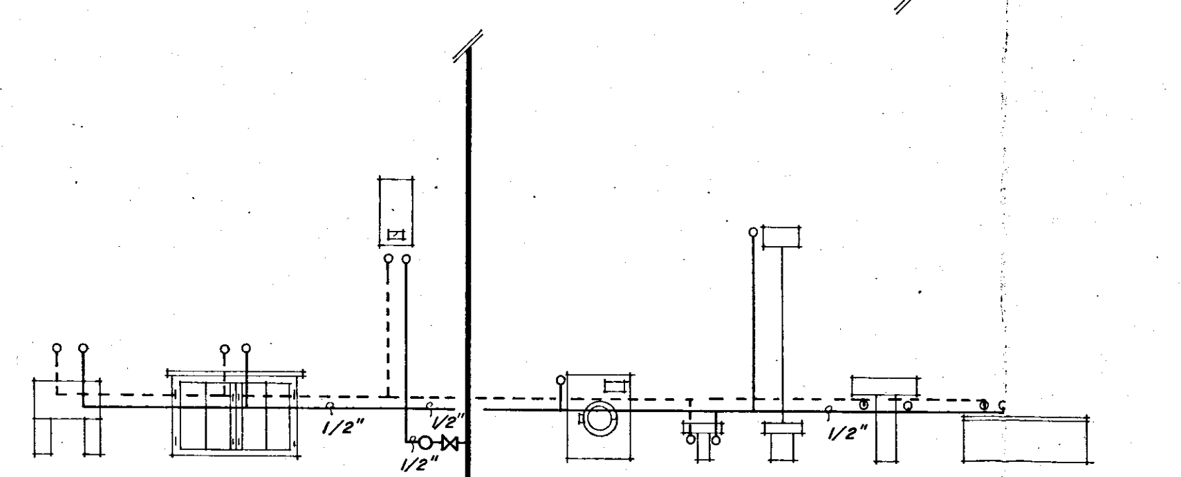
SCHEMA DISTRIBUZIONE IDRICA APP. DA 45
