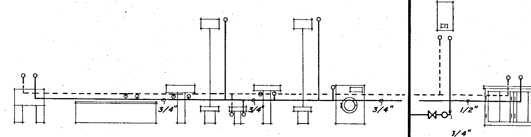
SCHEMA DISTRIBUZIONE IDRICA APP. DA 95 m
