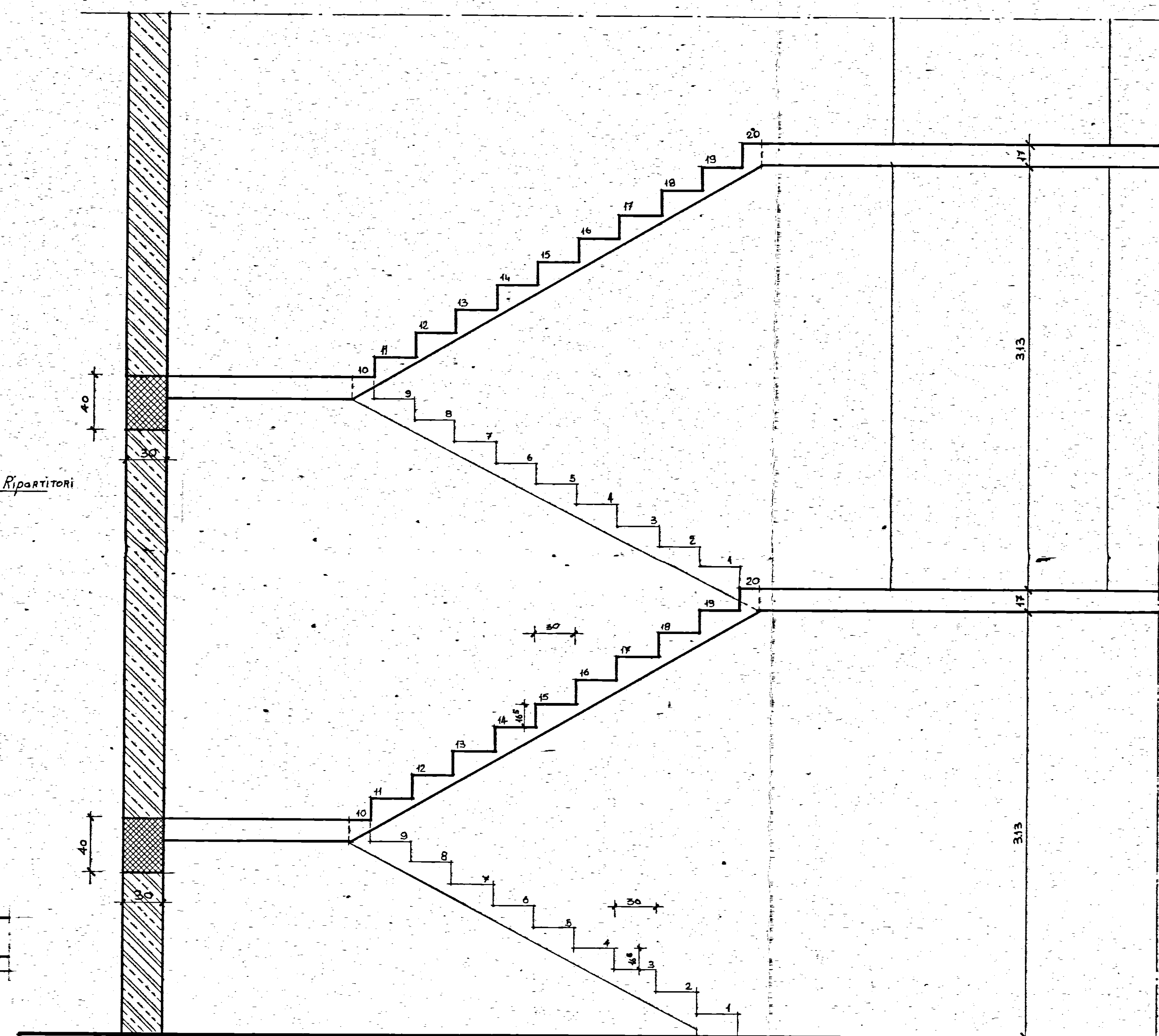
SEZIONE A-B
