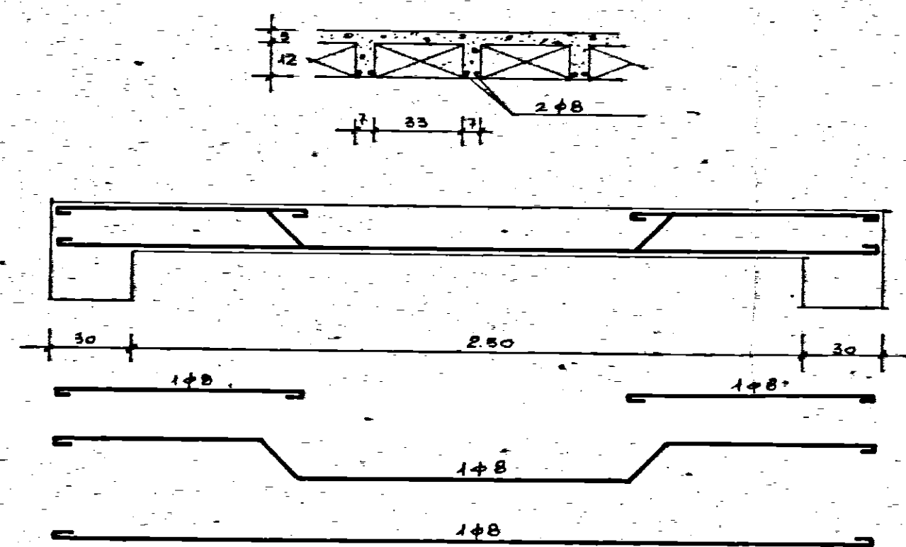
PARTICOLARE SOLAIO (A)
