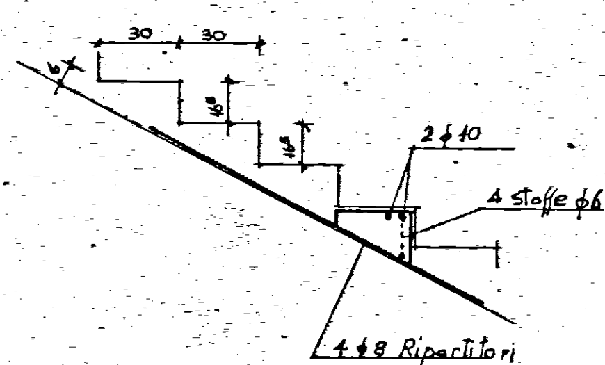
PARTICOLARE GRADINO
