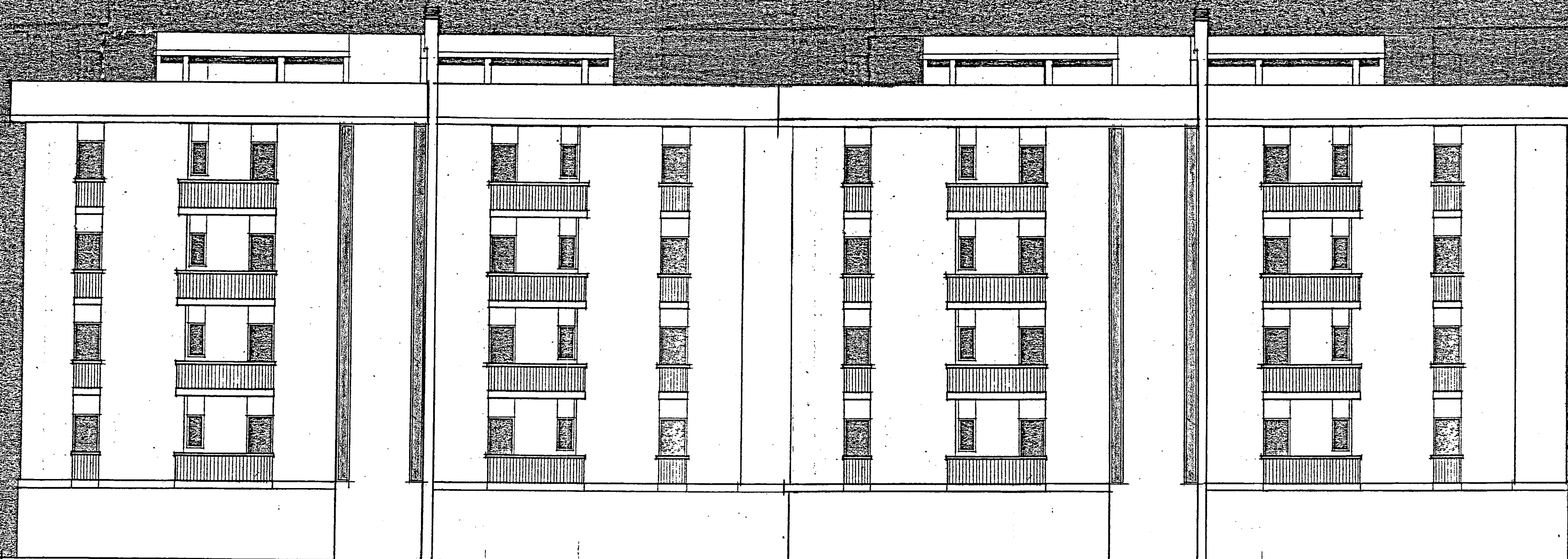
PROSPETTO POSTERIORE
