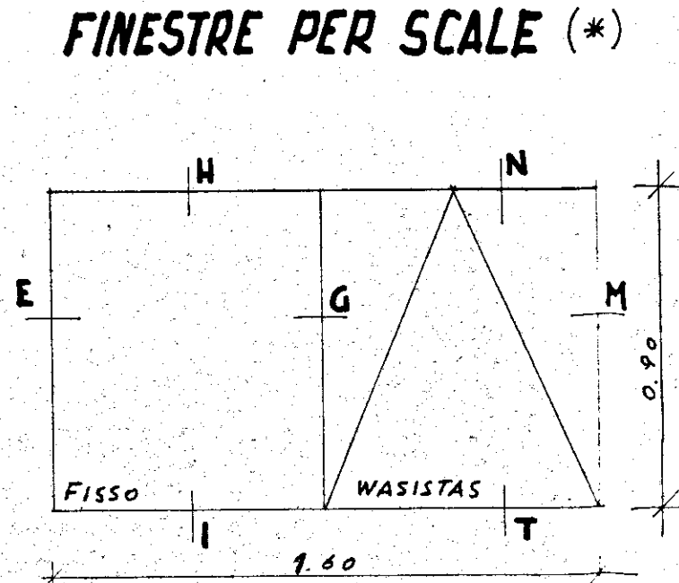
FINESTRA CON FISSO+WASISTAS, TIPO F7 PER SCALE
