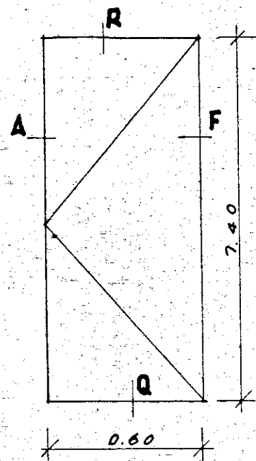
FINESTRA TIPO F5 CON AVVOLGIBILE
