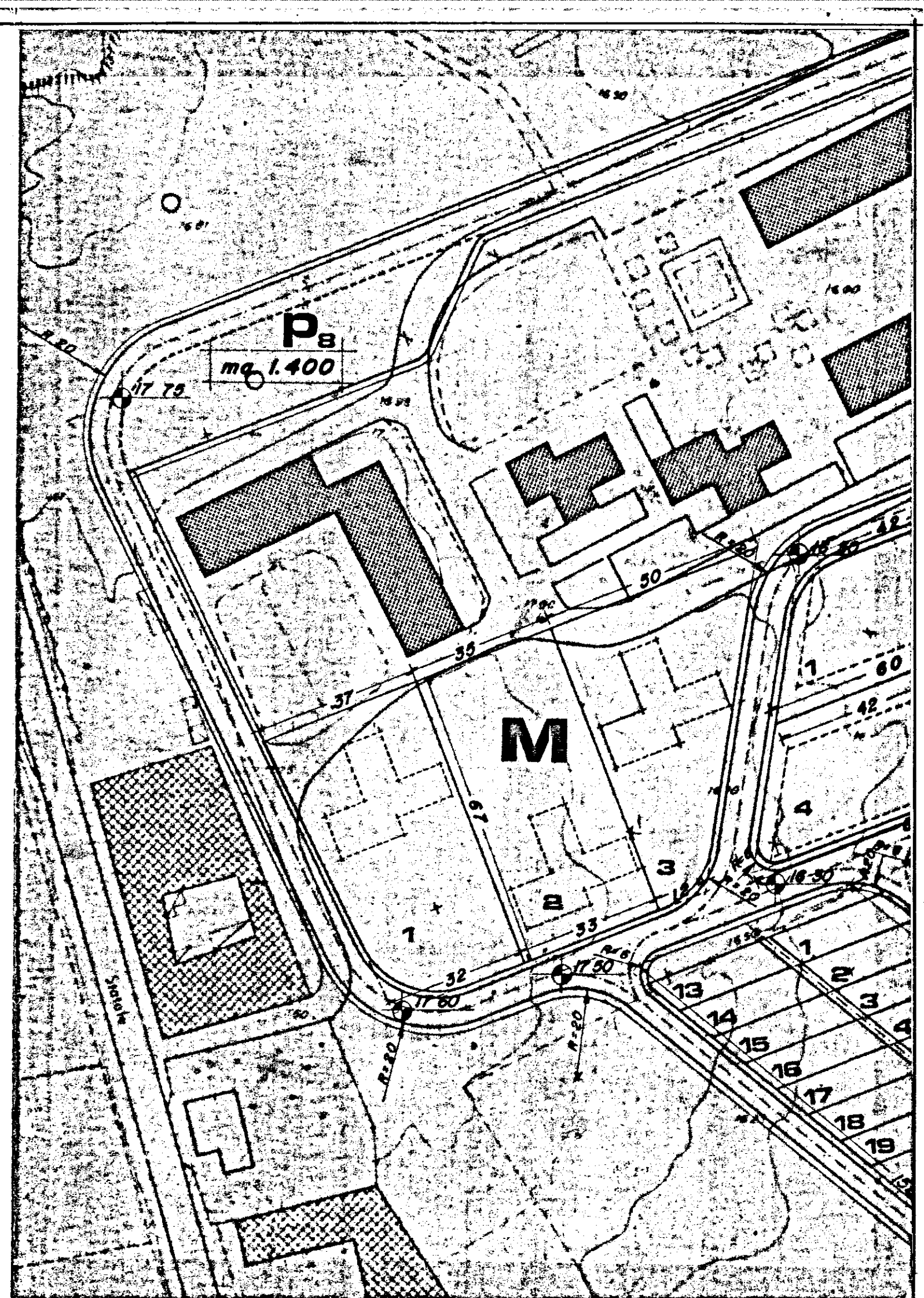
STRALCIO PLANIMETRICO DEL PIANO DI ZONA DEL RIONE PERRINO 1: 1000
