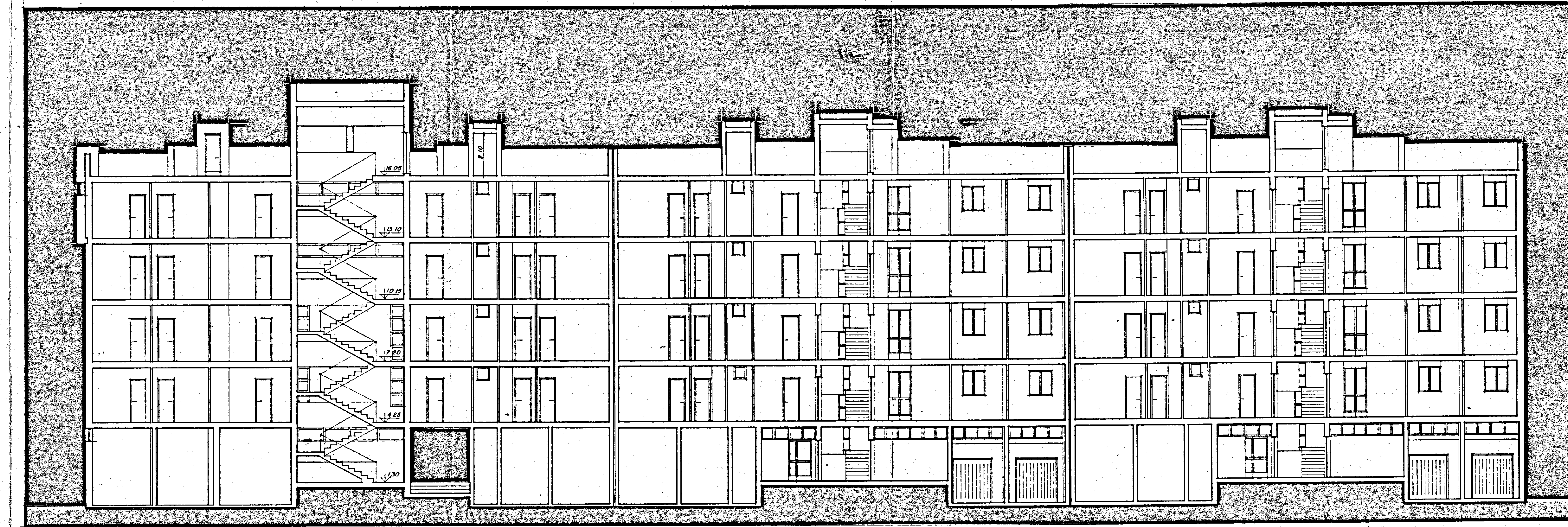
SEZIONE X-X
