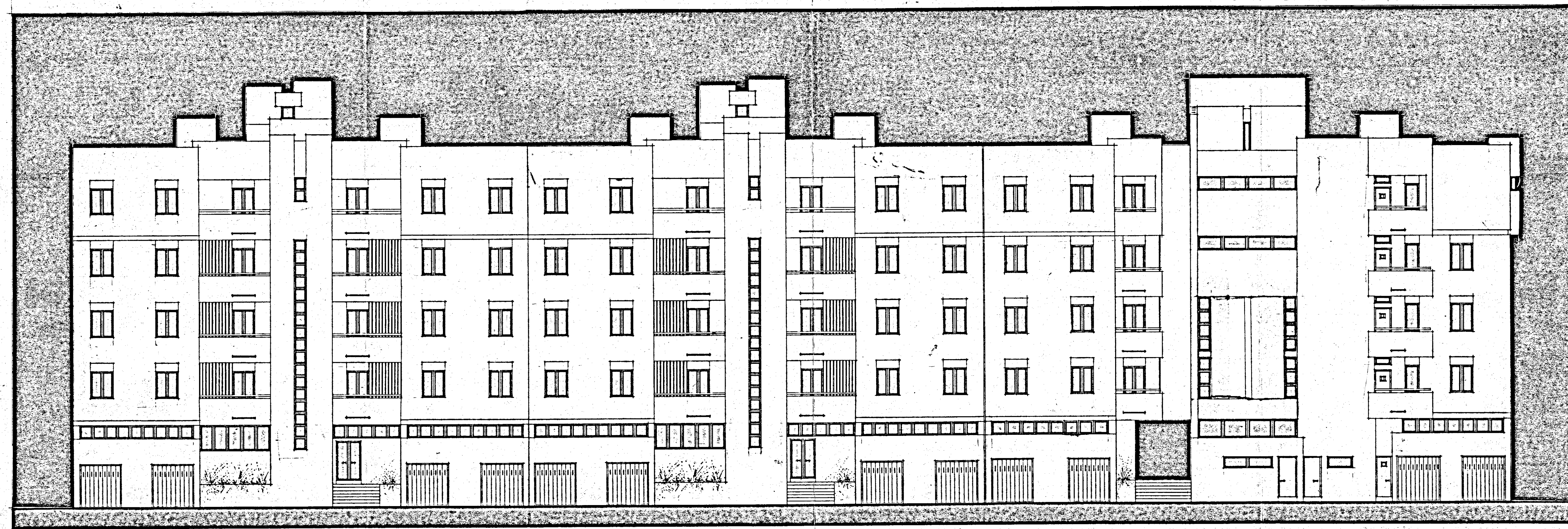
PROSPETTO - C -
