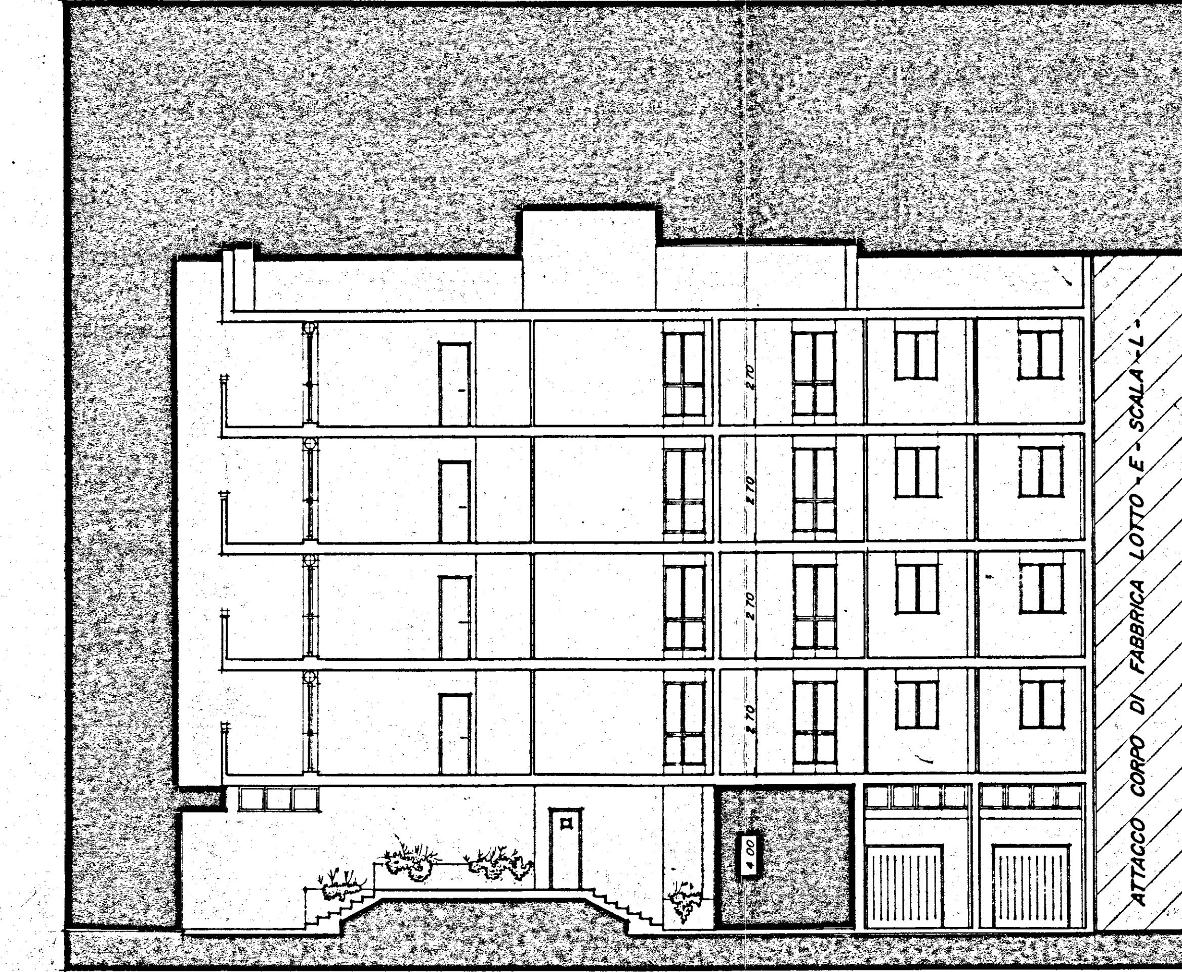
SEZIONE Y-Y
