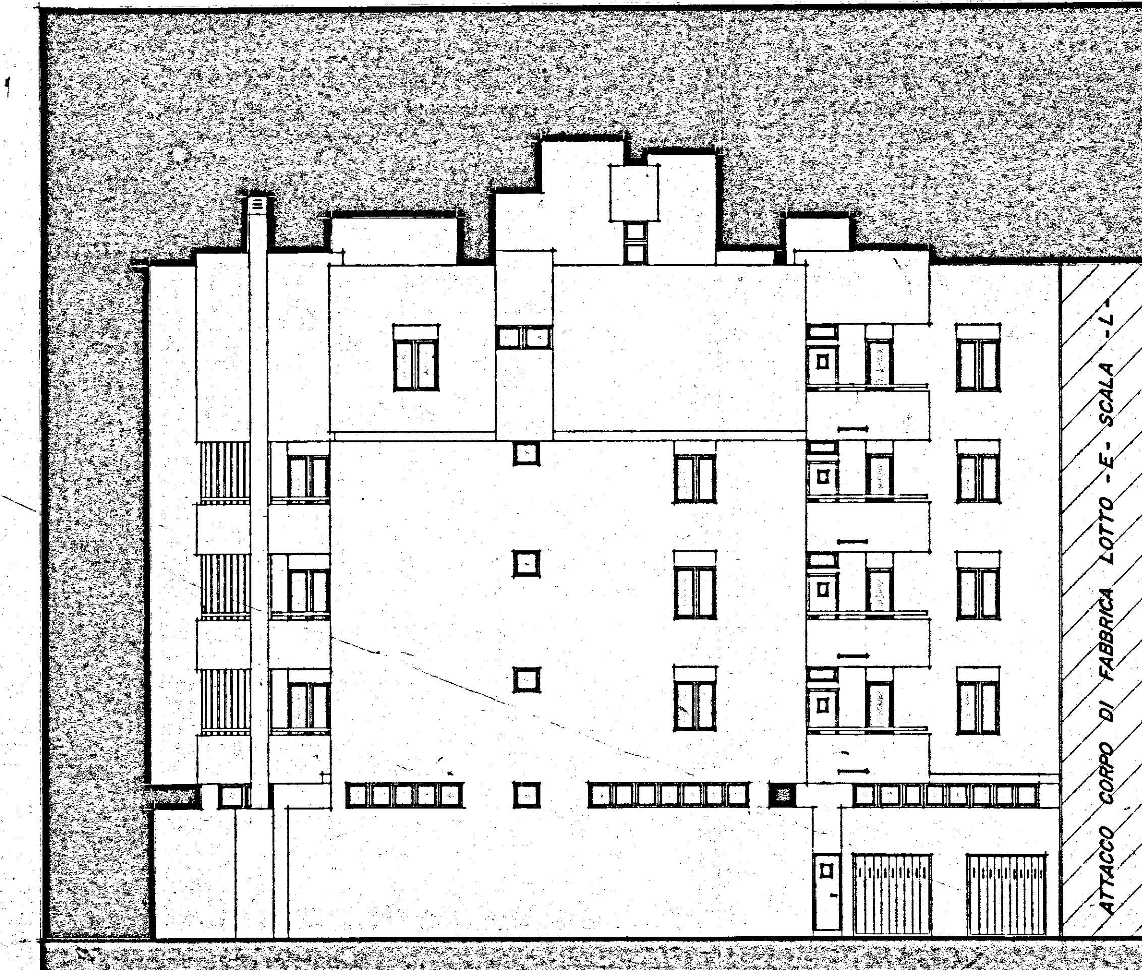
PROSPETTO - D -
