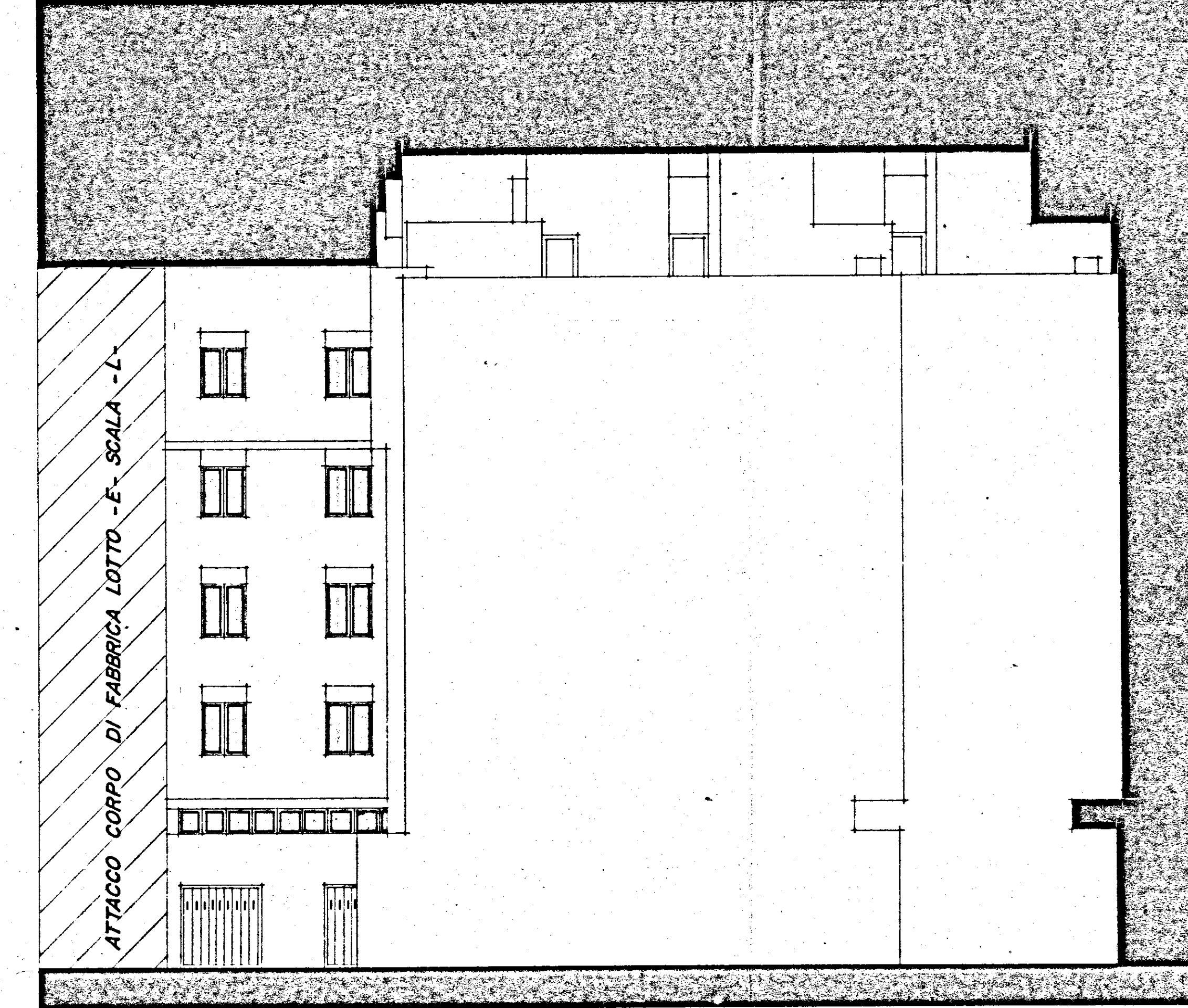
PROSPETTO - B -
