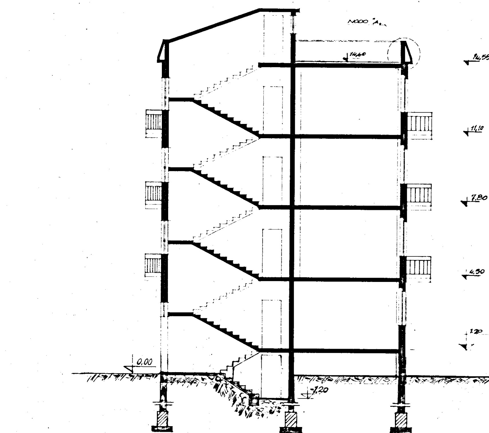
SEZIONI X-X
