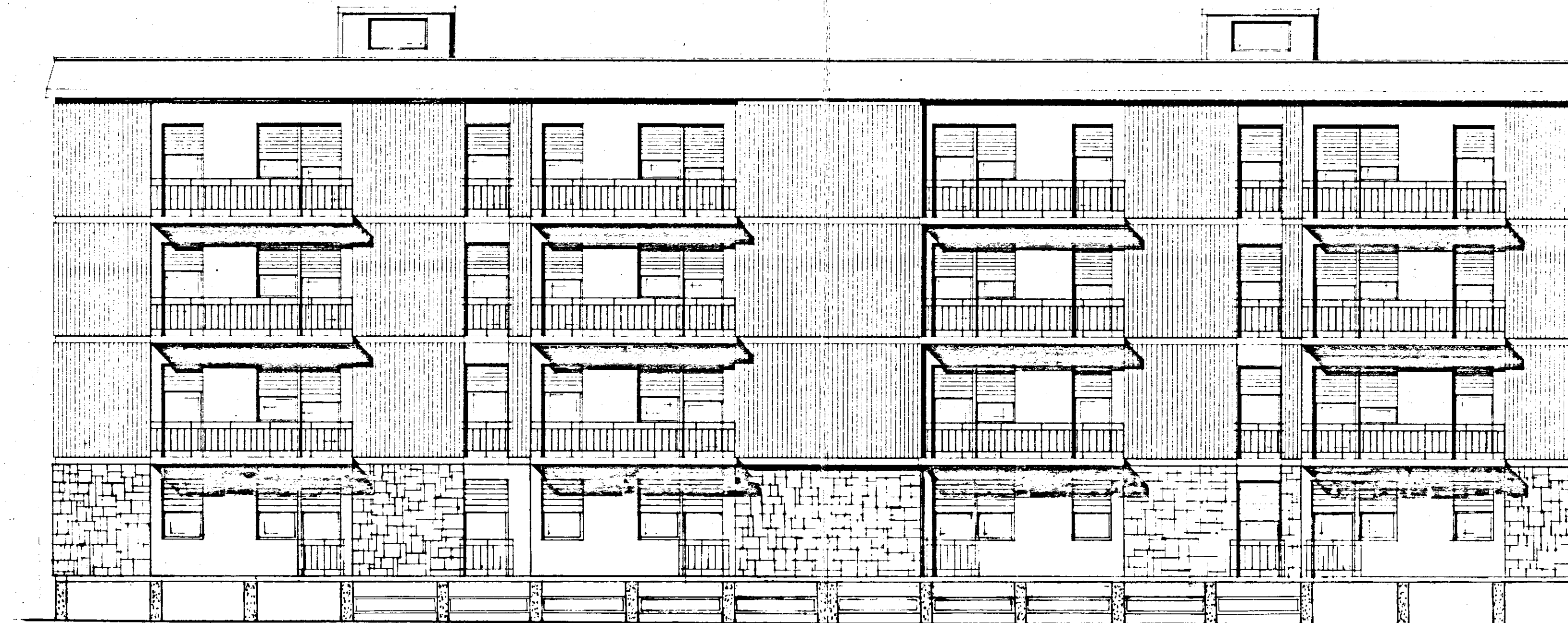
PROSPETTO "C"
