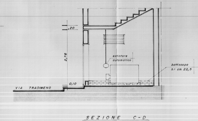
SEZIONE C-D
