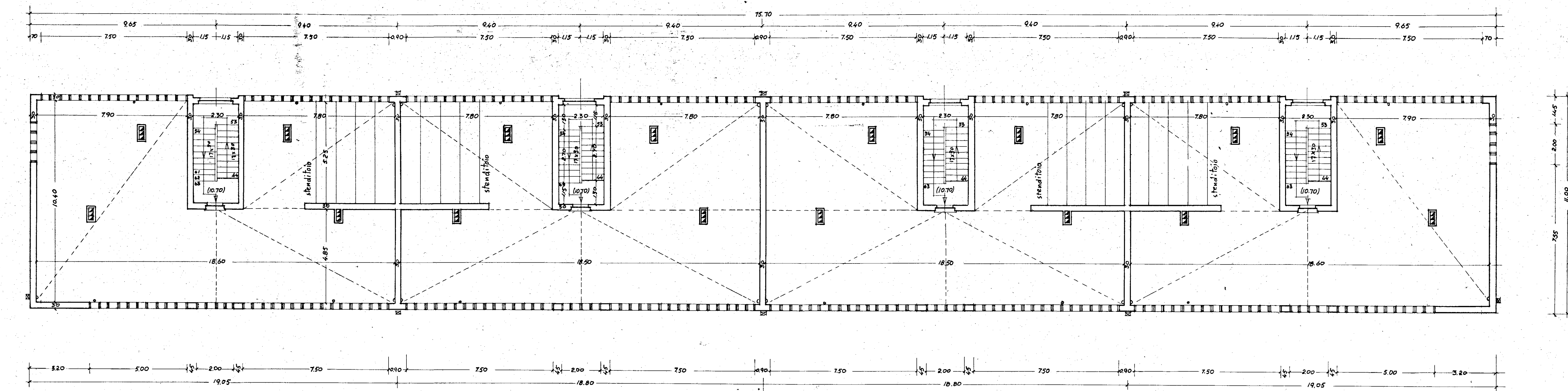
DIS. N° 176 PIANTA COPERTURA RAPP. 1:100
