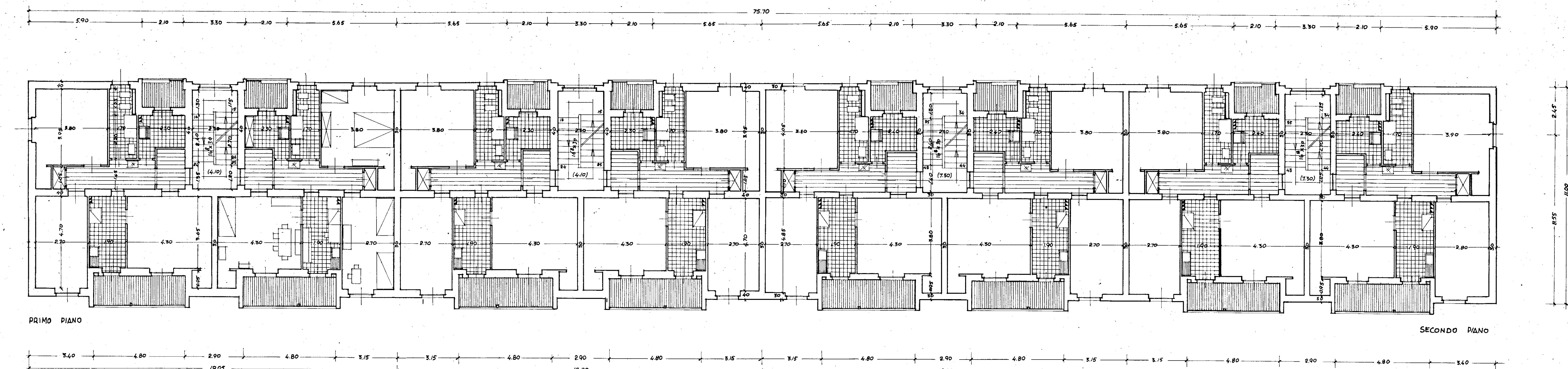
DIS. N° 175 PIANO TIPO (I° E II°) RAPP. 1:100
