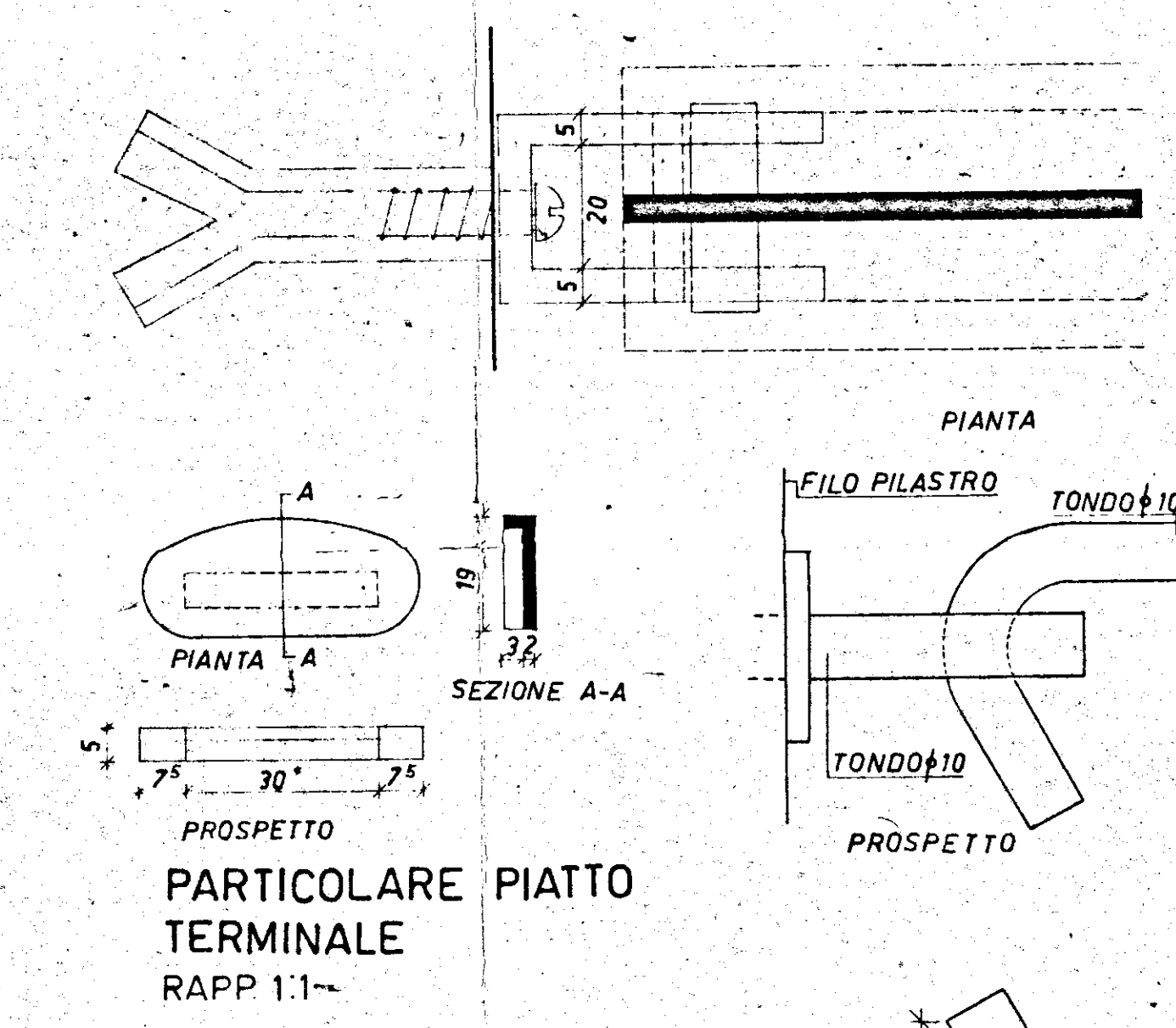
PARTICOLARE ATTACCO DEL TONDO AL PILASTRO RAPP. 1:1
