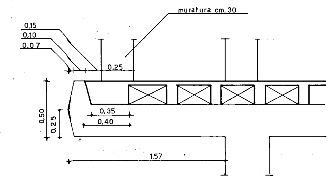
Sezione A - A rapp. 1:20
