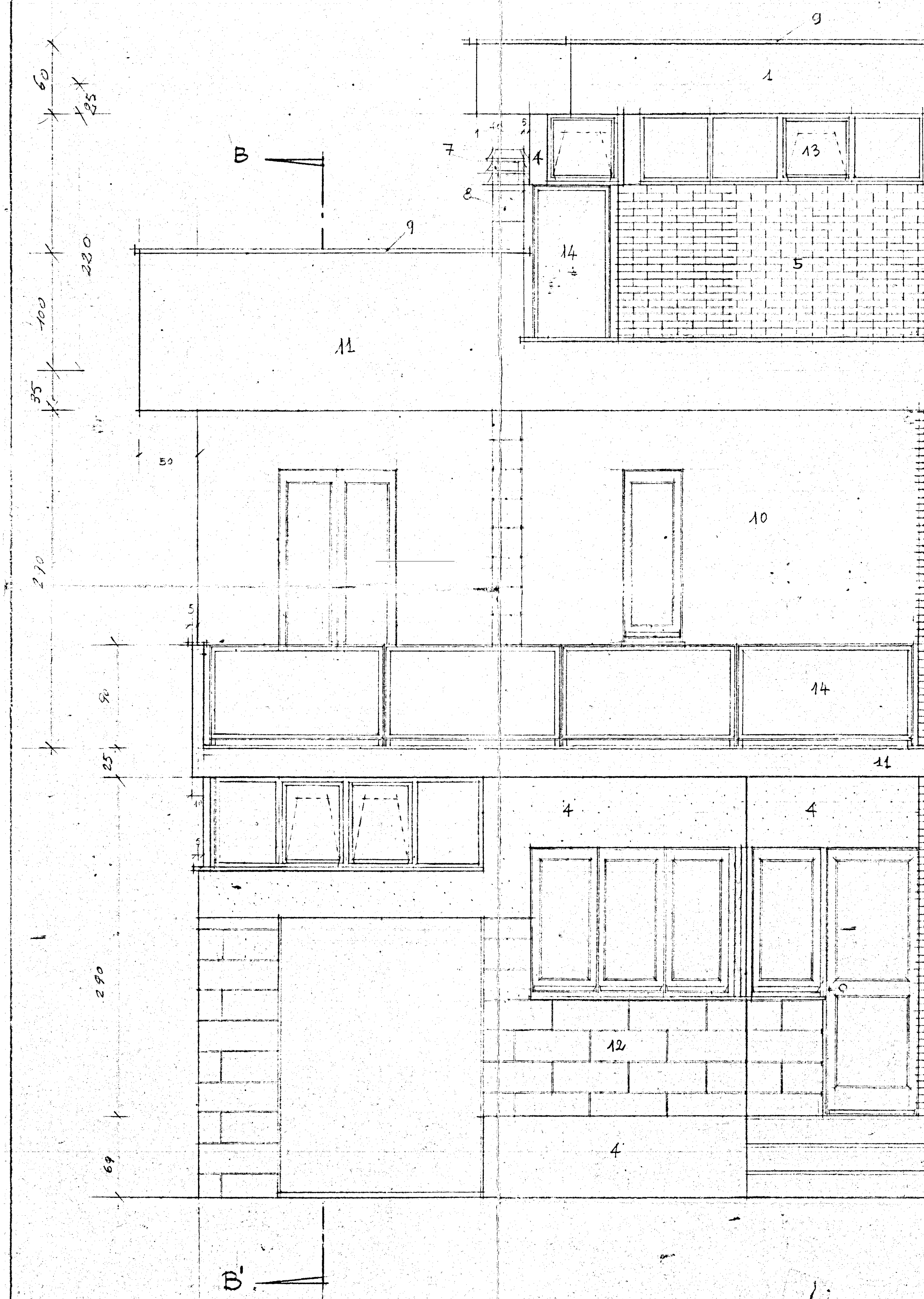
PROSPETTO "B" (GARAGE E INGR. CUCINA)
