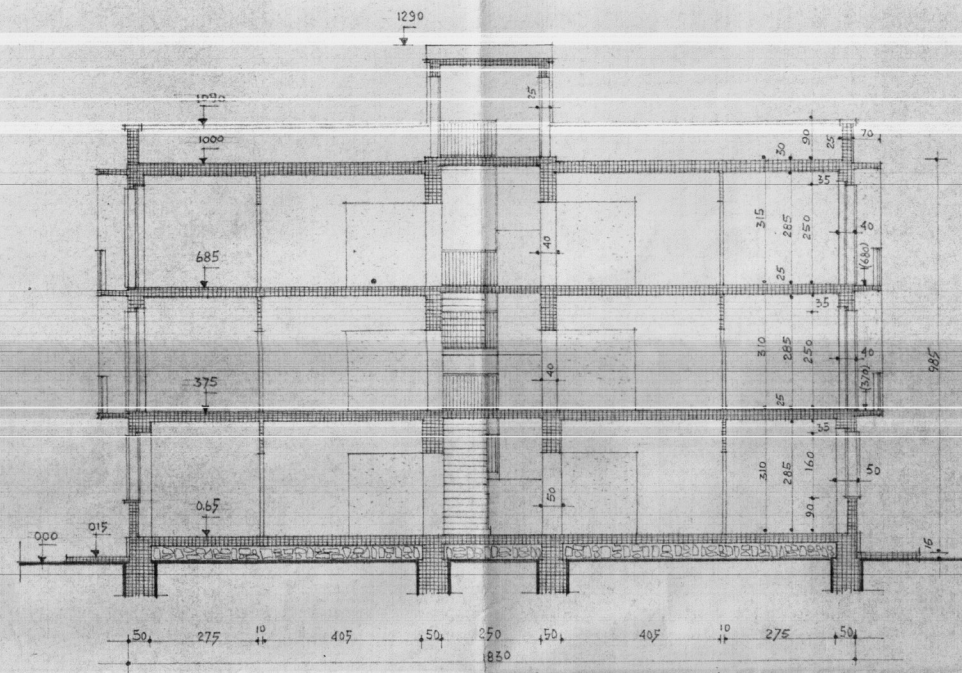
• SEZIONE C-D • RAPP. 1:100 •
