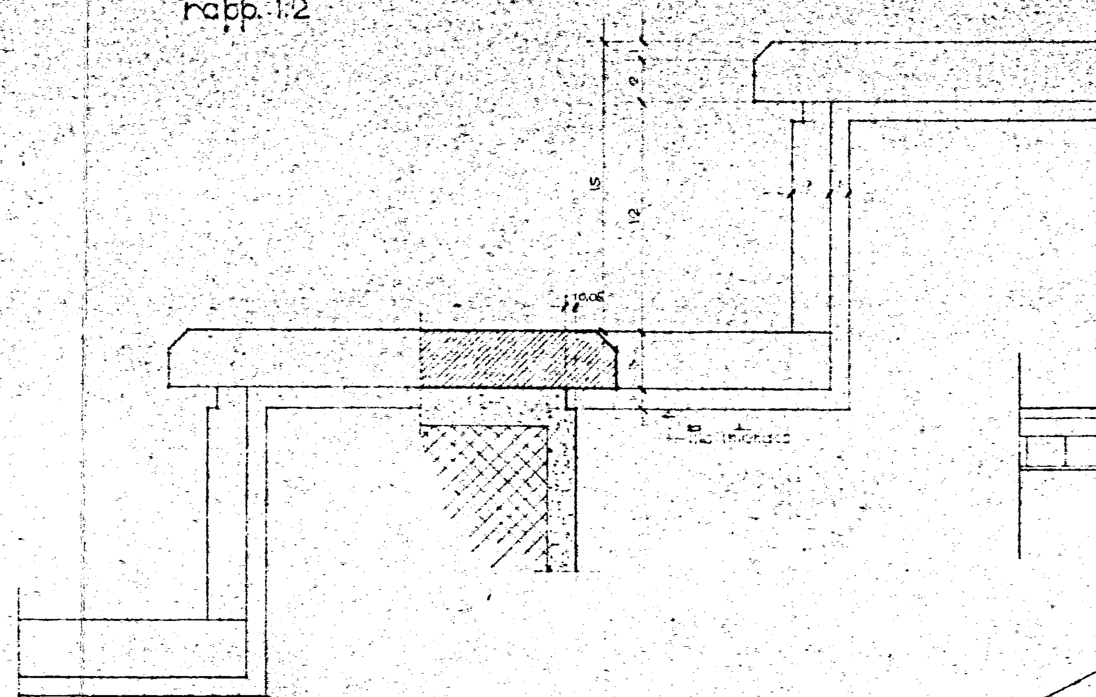
PARTICOLARE GRADINO rapp. 1:2
