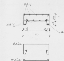
SEZIONE TRAVE DI CORONAMENTO PORTICO RAPPO 1:20
