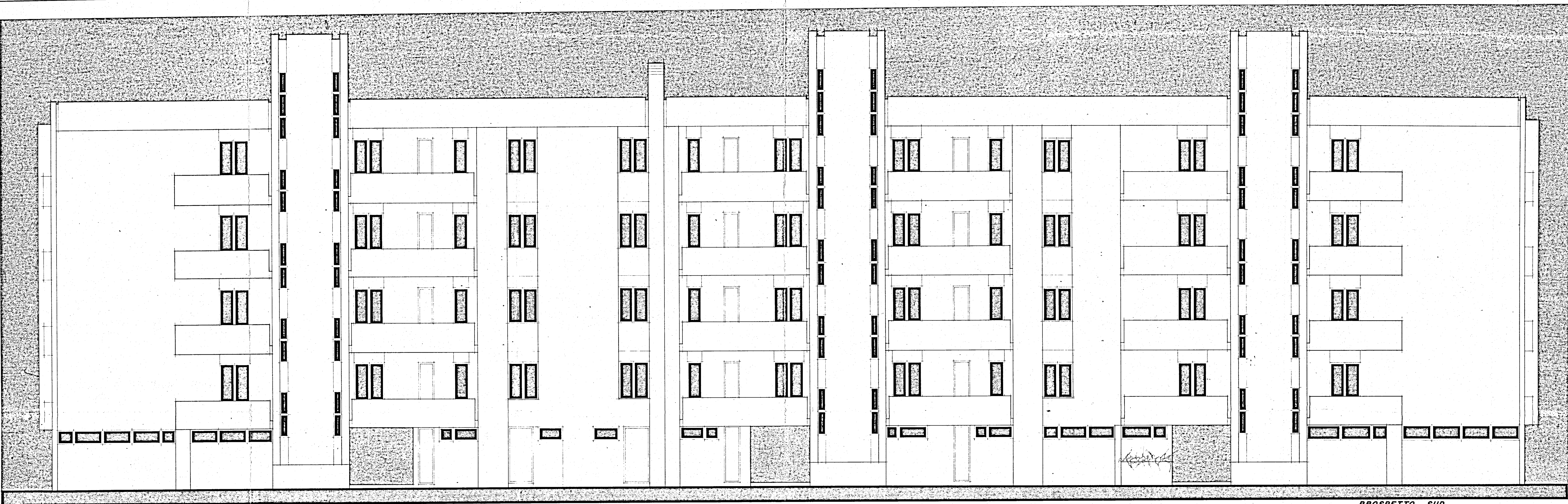
PROSPETTO SUD
