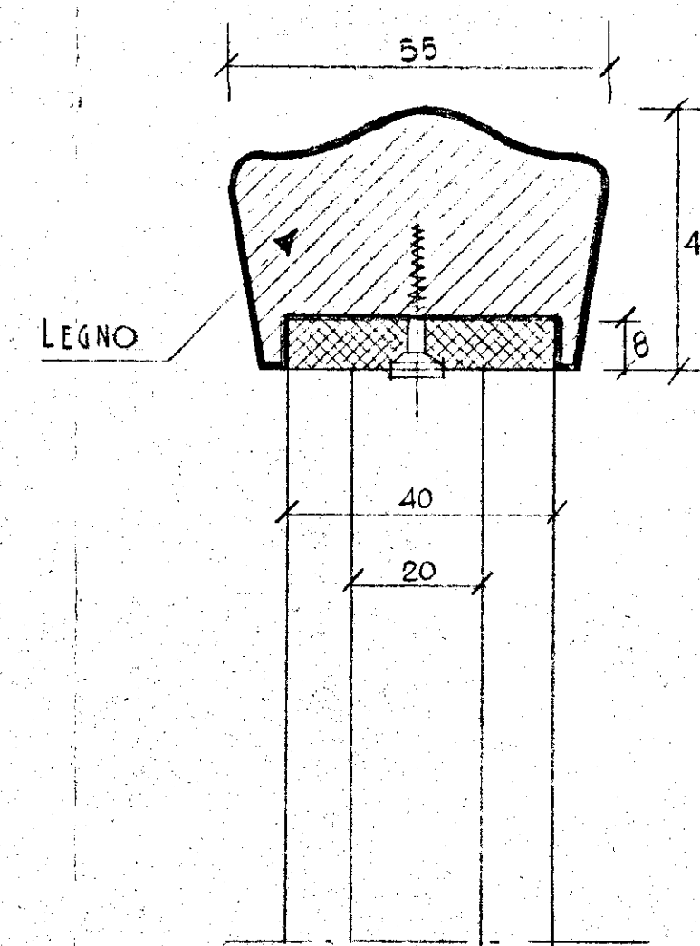
CORRIMANO - RAPP. AL VERO
