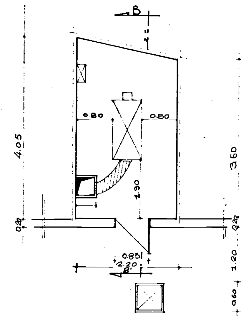
RILIEVO PIANTA CENTRALE TERMICA
