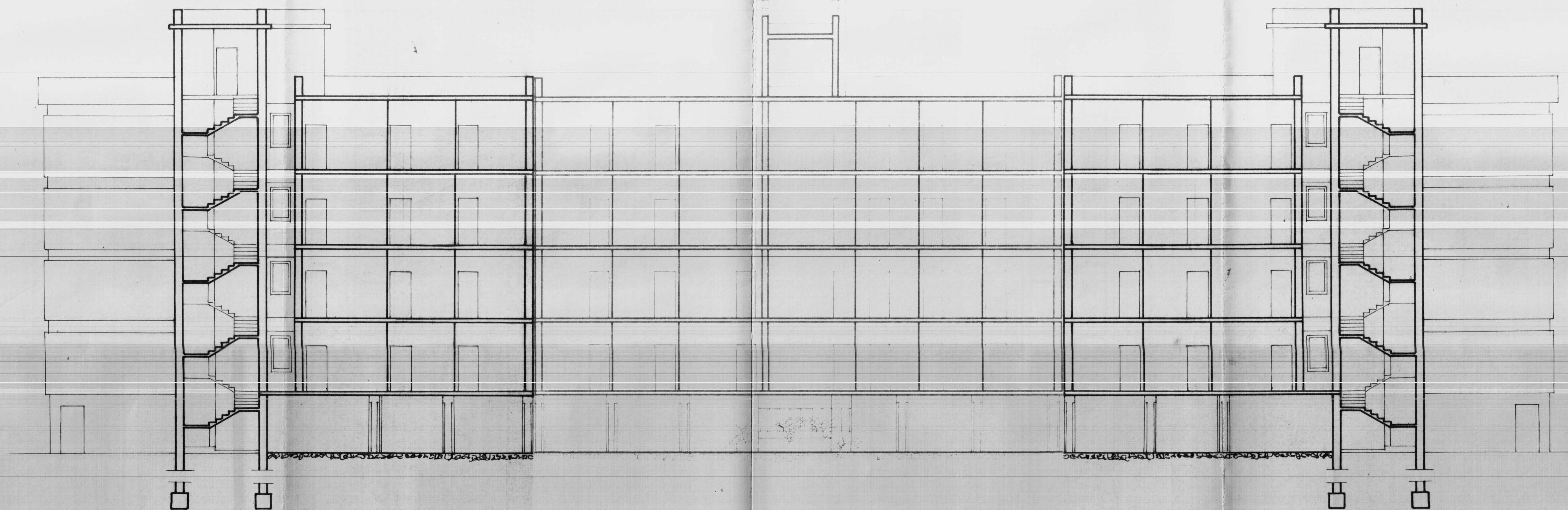
SEZIONE 'C.C.'
