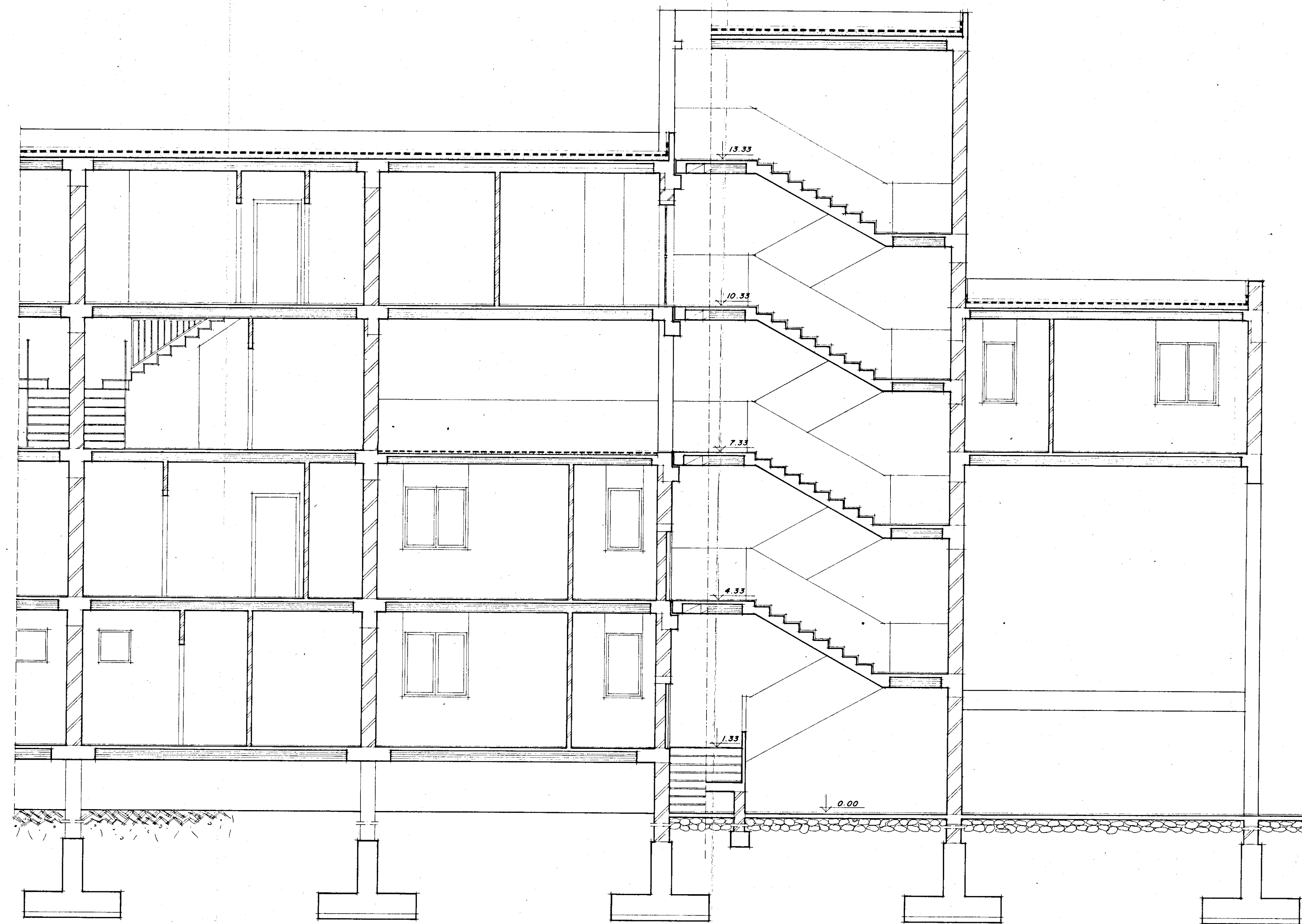
SEZIONE Z-Z
