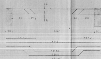
TRAVE T.1
