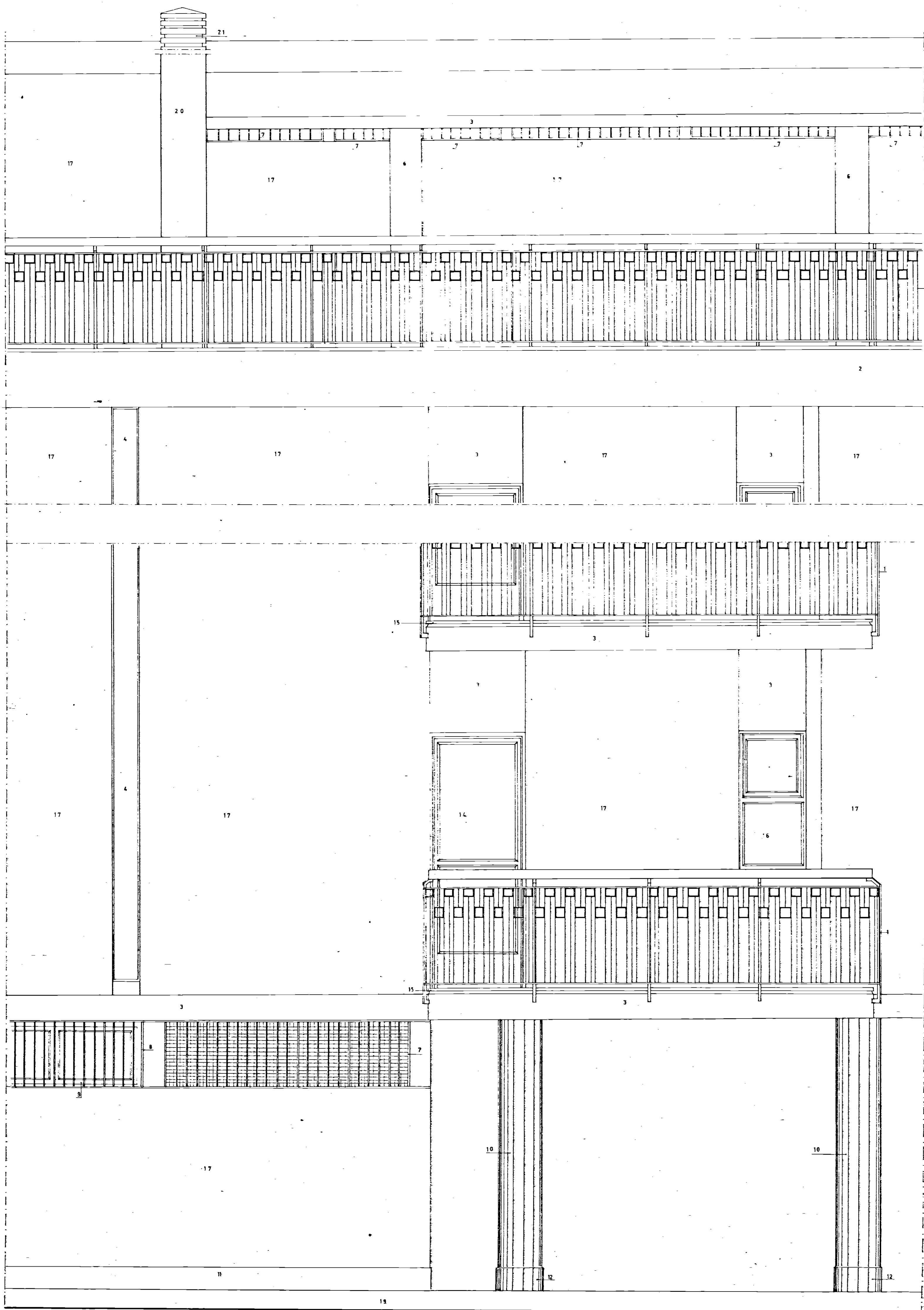
PROSPETTO POSTERIORE
