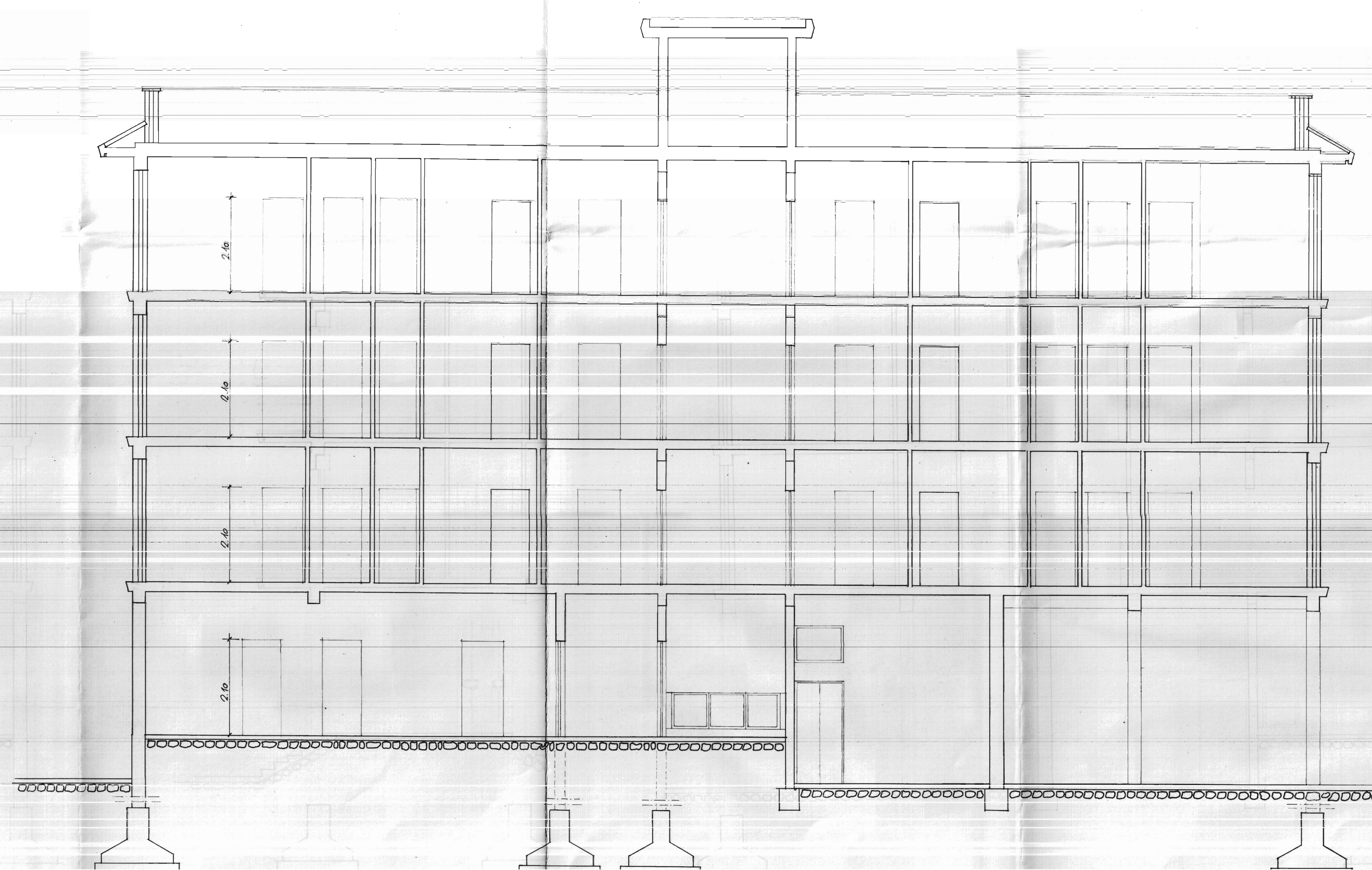
- SEZIONE c-c -
