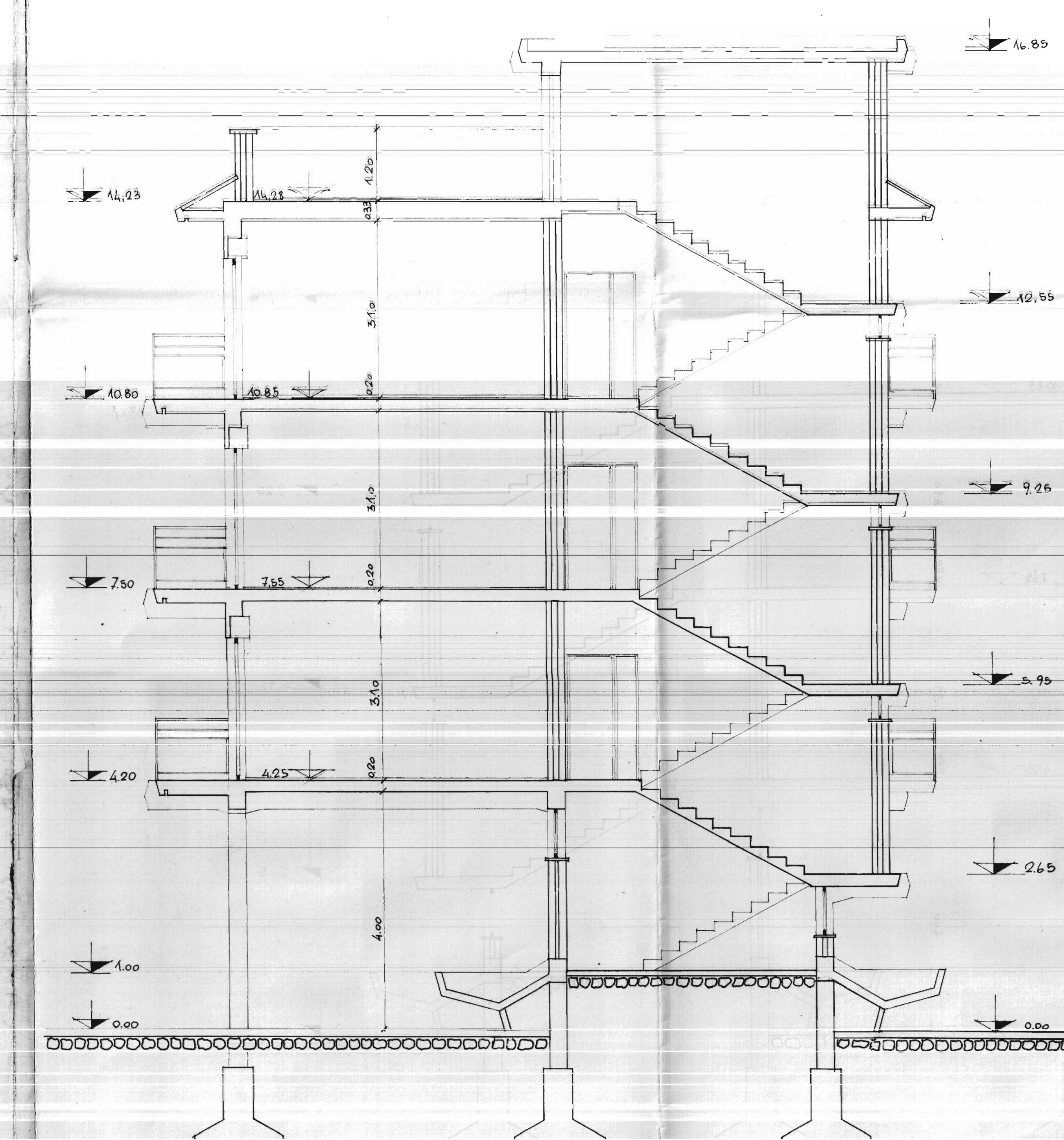
- SEZIONE d-d -
