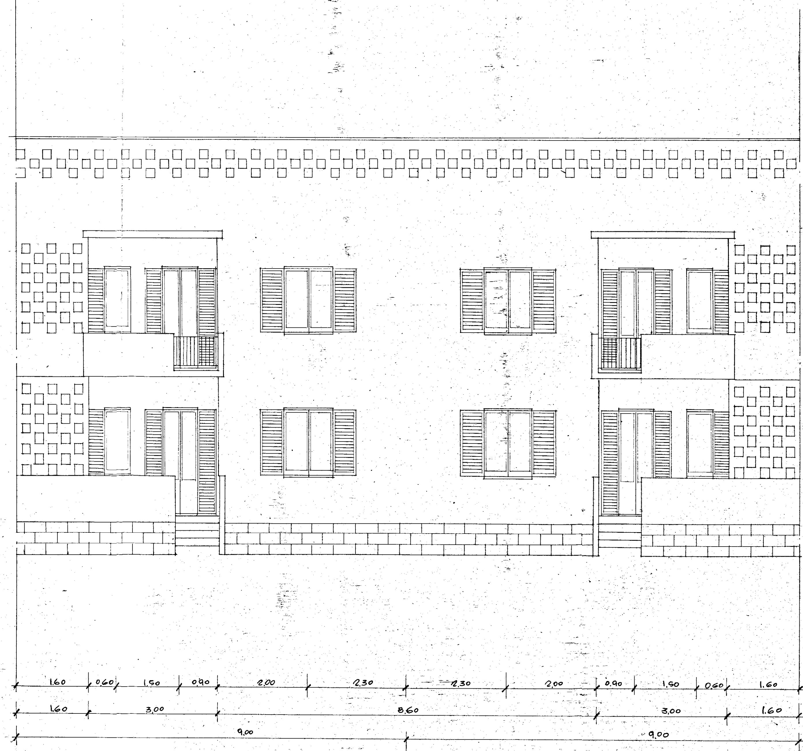
DIS. N° 144 PROSPETTO OVEST (PARTICOLARE DEL PROSPETTO A TAG N° 55) RAPP. 1:50
