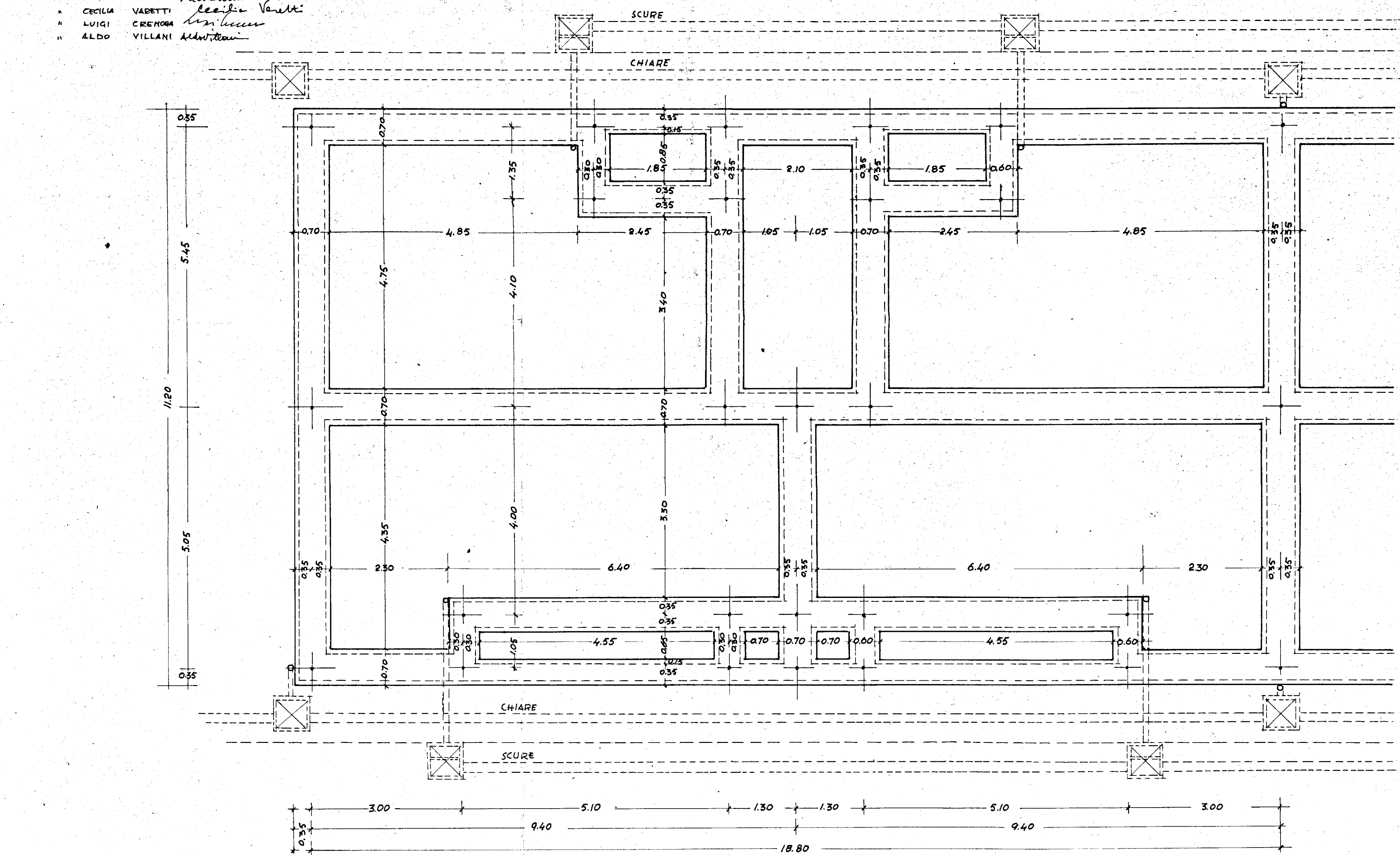
DIS. N° 179 PIANTA FONDAZIONE (PARTICOLARE DELLA PIANTA A TAV. 72) RAPP. 1:50
