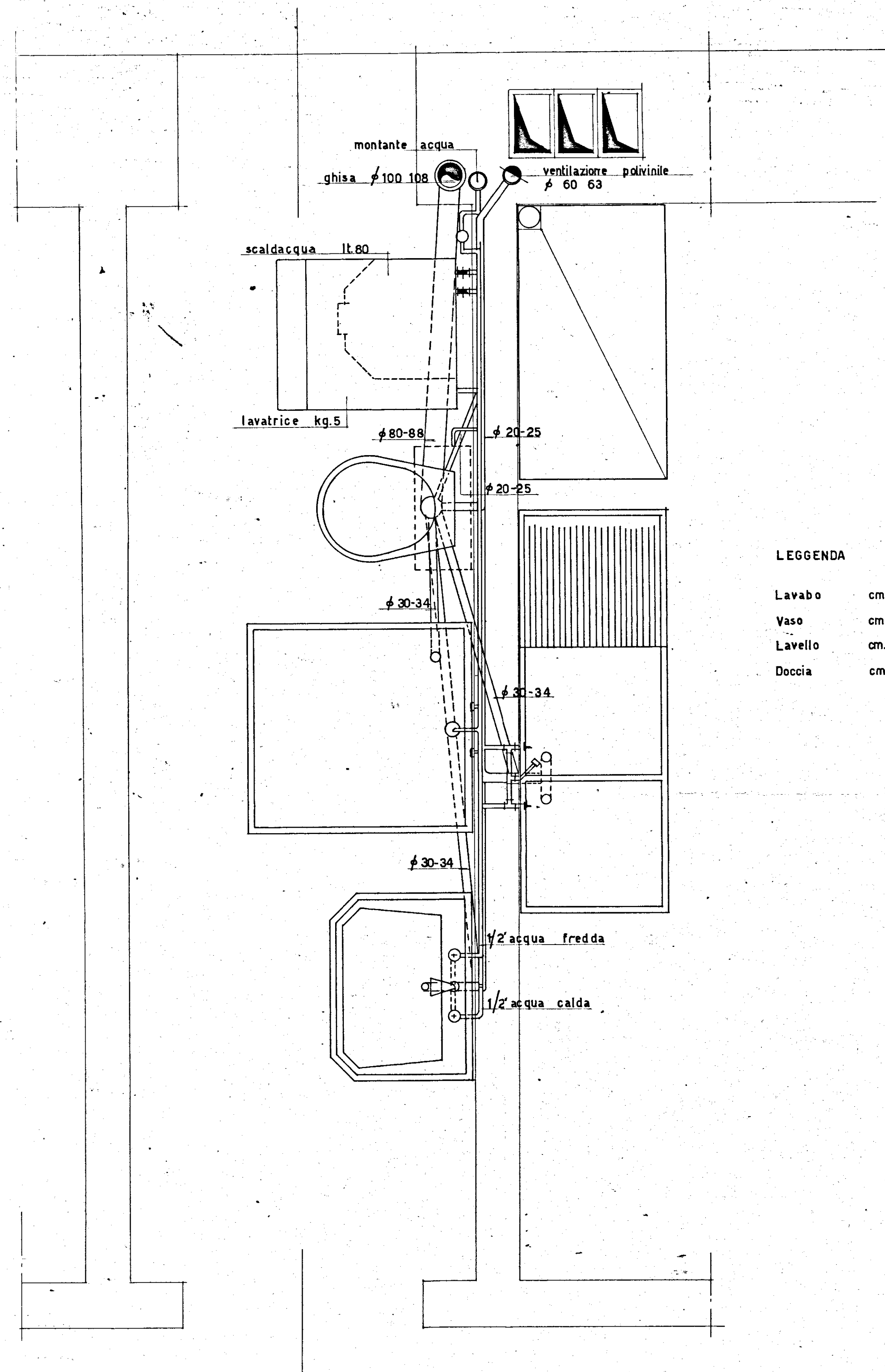
PIANTA Rapp. 1:10
