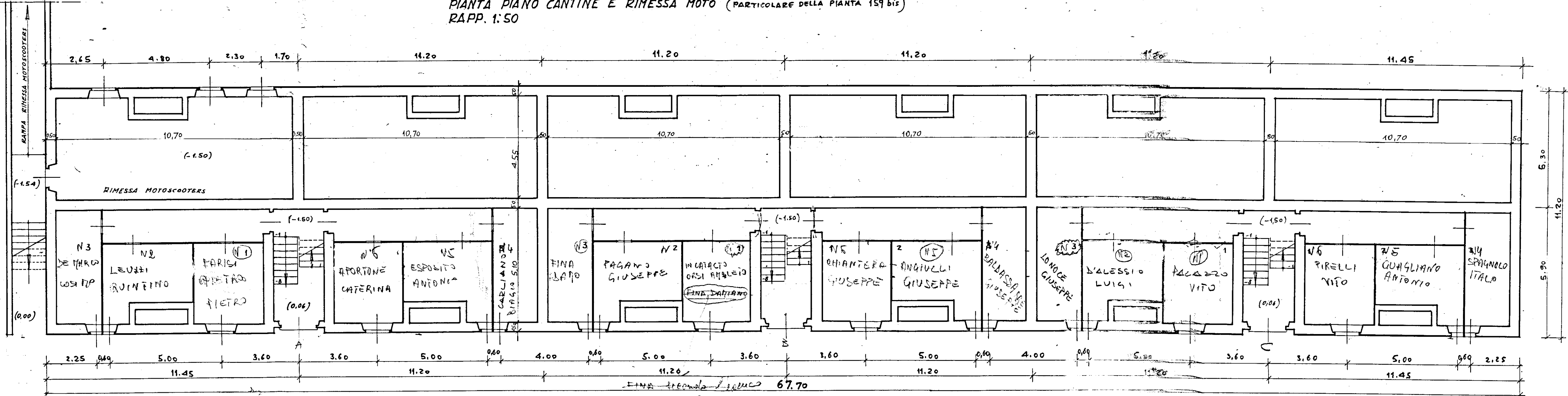
DIS. N° 159 bis PIANA PIANO CANTINE RAPP. 1:100
