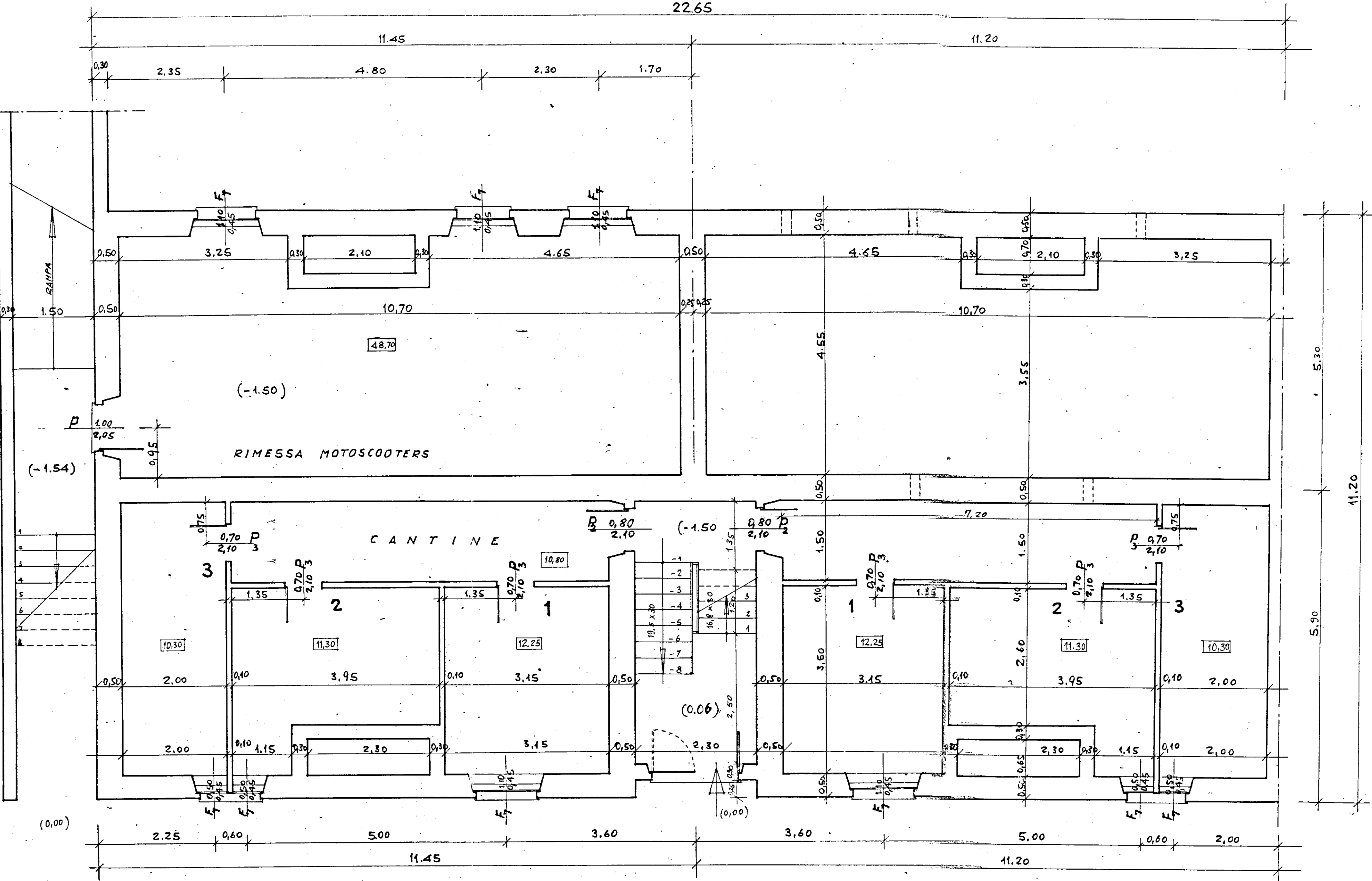
DIS. N° 166 bis PIANA PIANO CANTINE E RIMESSA MOTO (PARTICOLARE DELLA PIANA 159 bis) RAPP. 1:50
