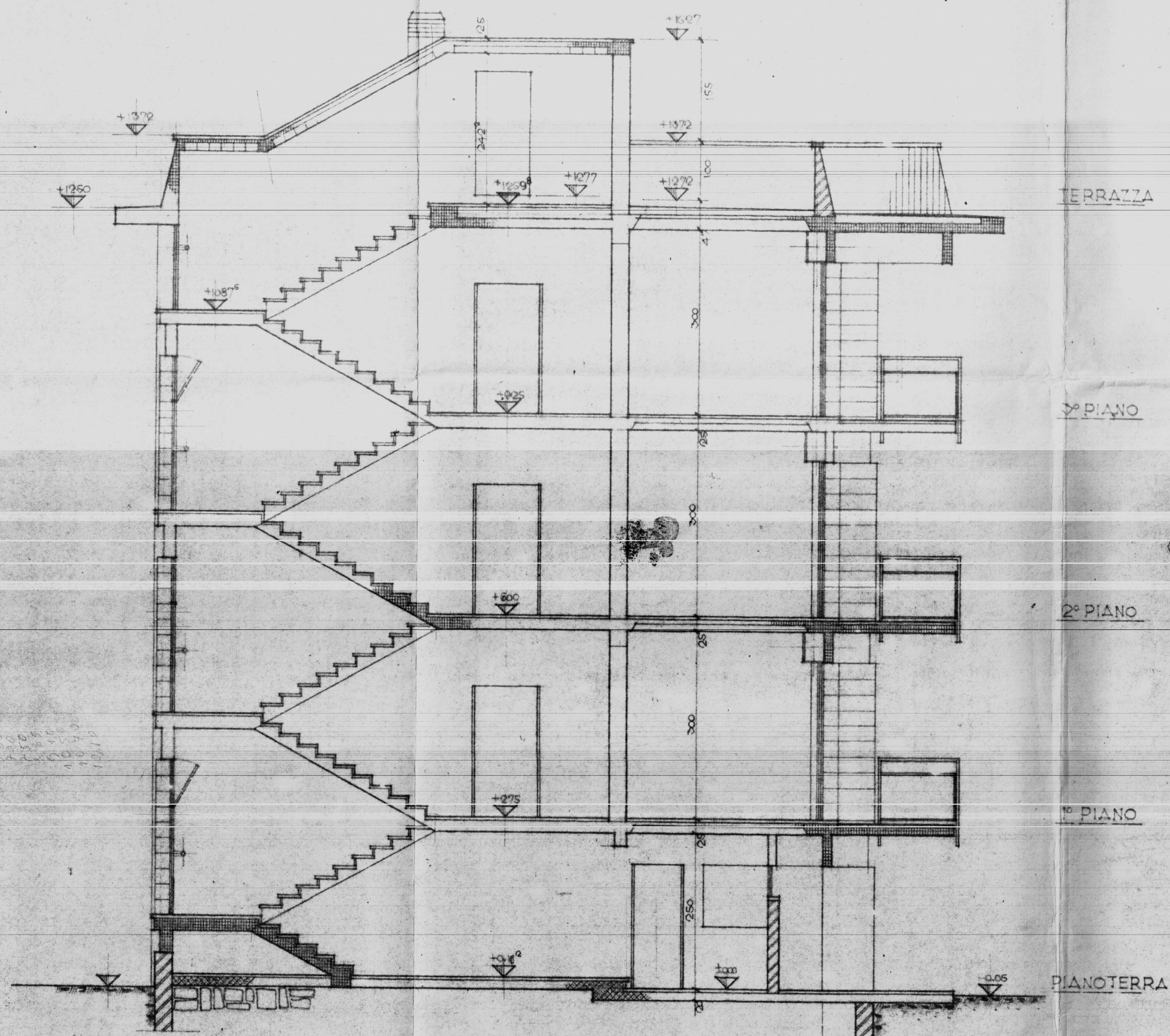
SEZIONE E-F
