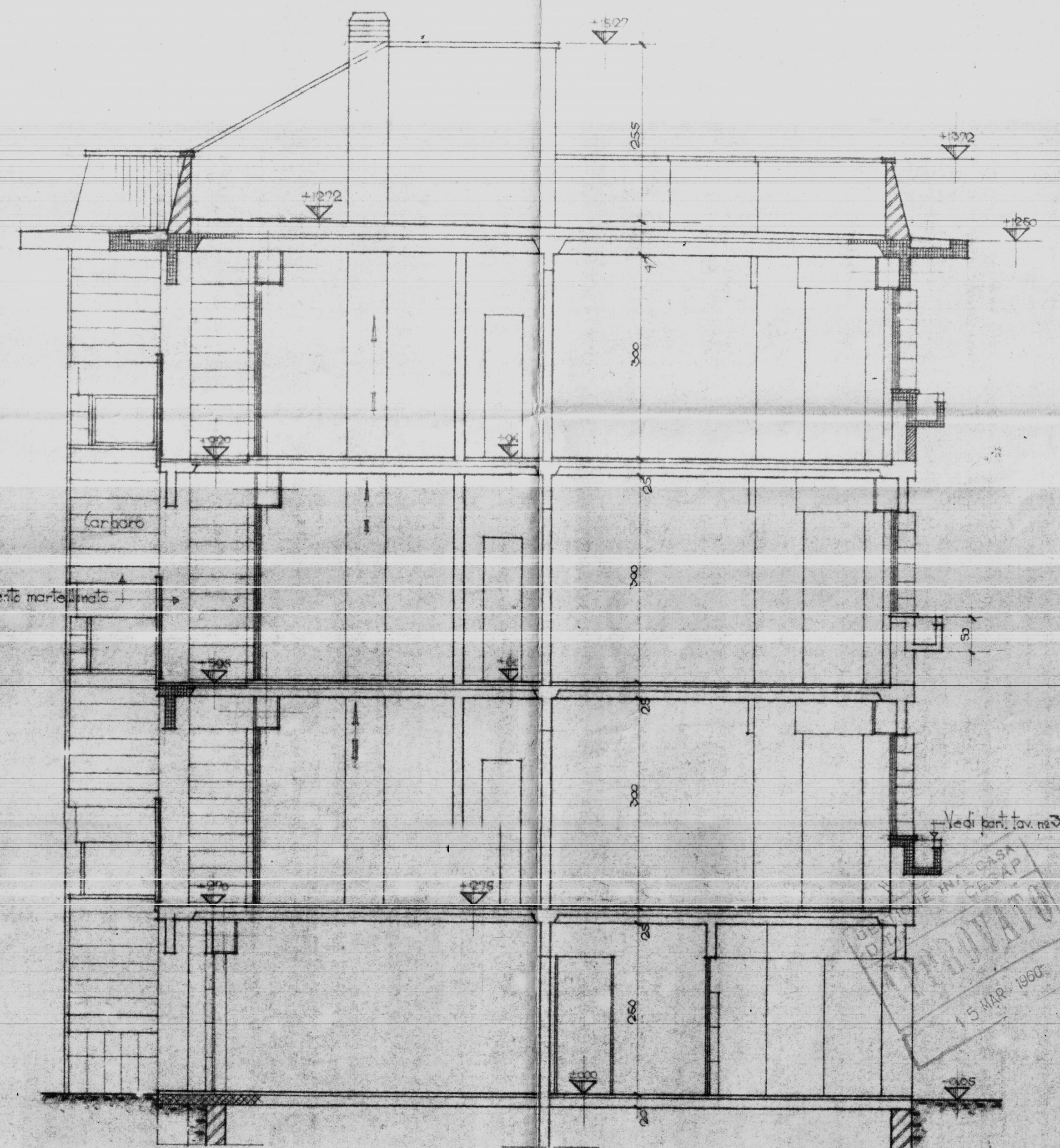
SEZIONE G-II
