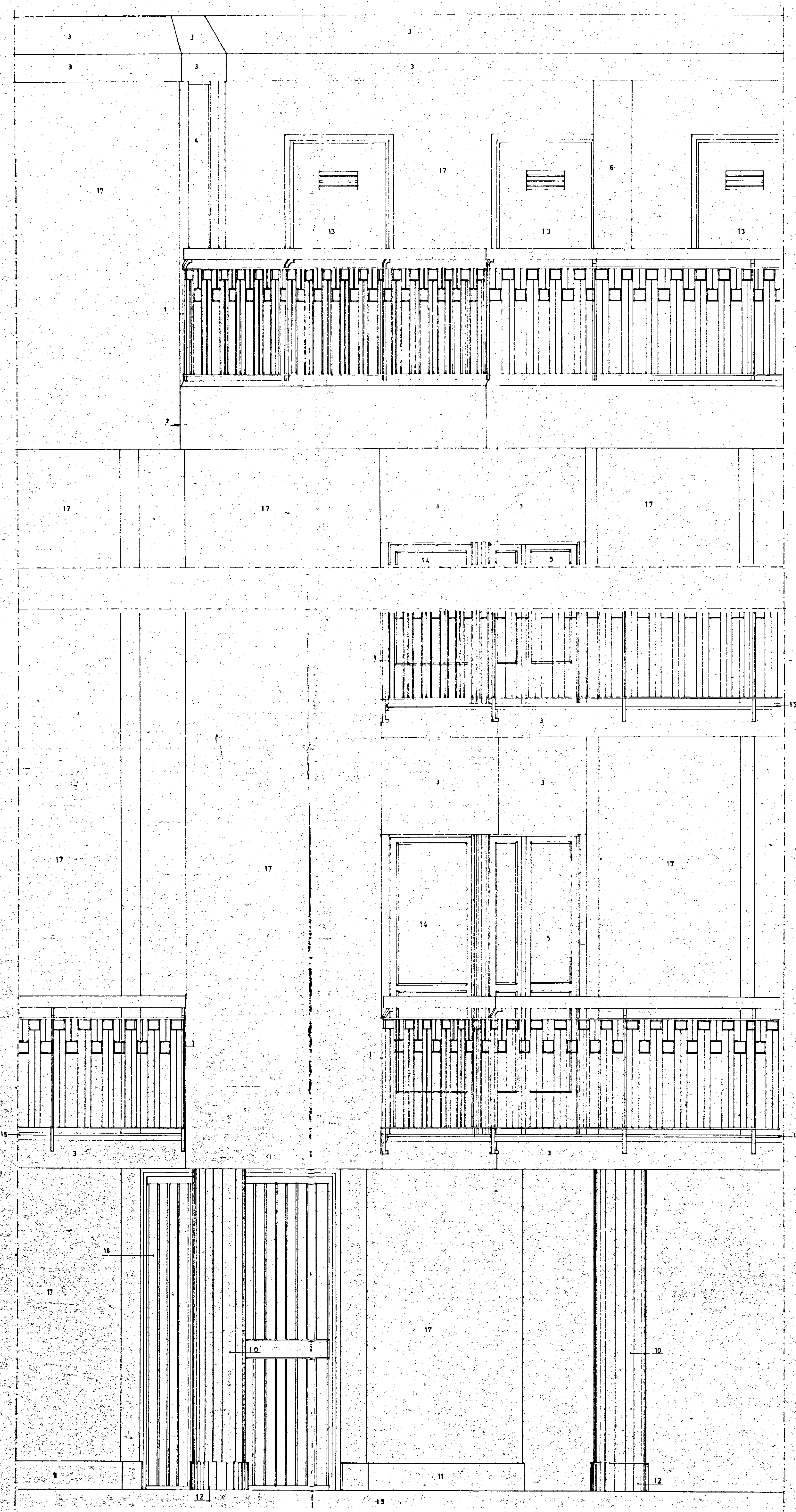
PROSPETTO ANTERIORE
