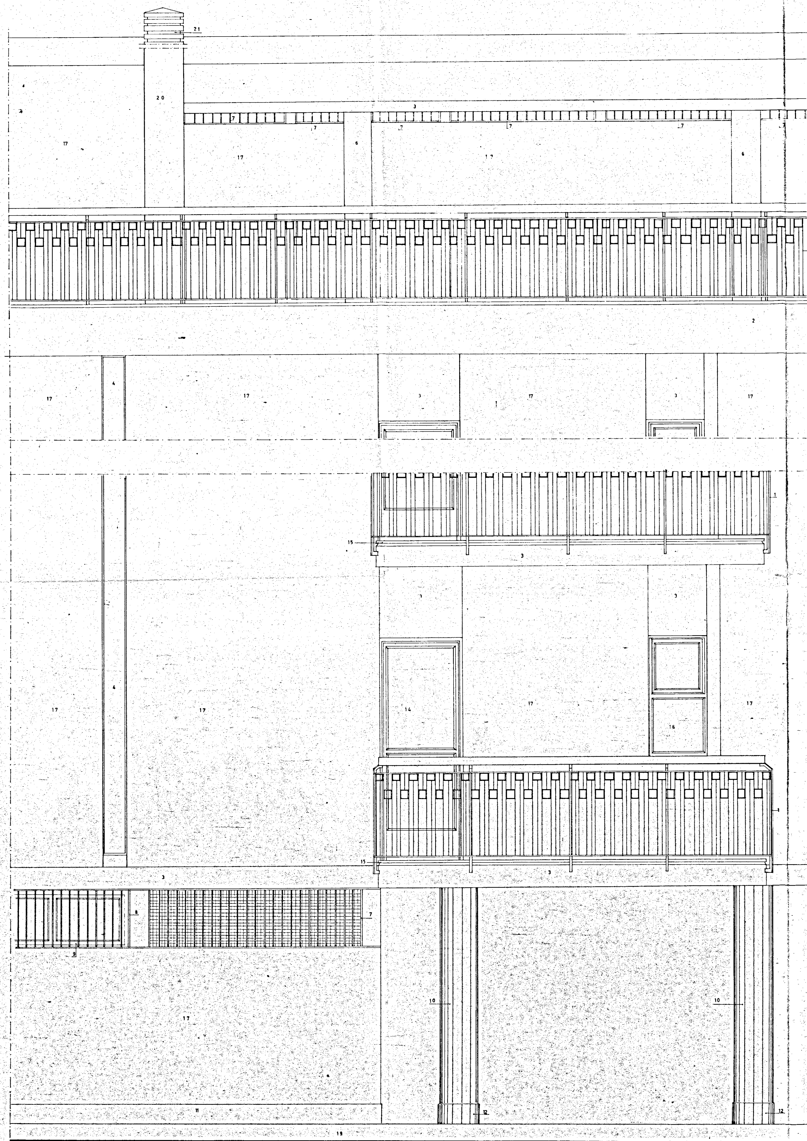
PROSPETTO POSTERIORE
