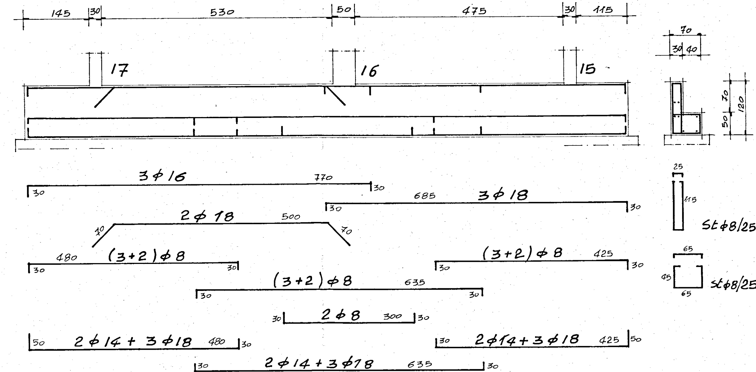
SEZ. A-B
