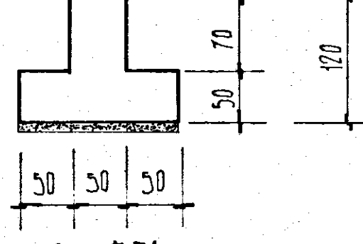
SEZ. E-E'
