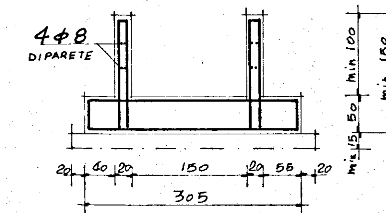
SEZ. A-B
