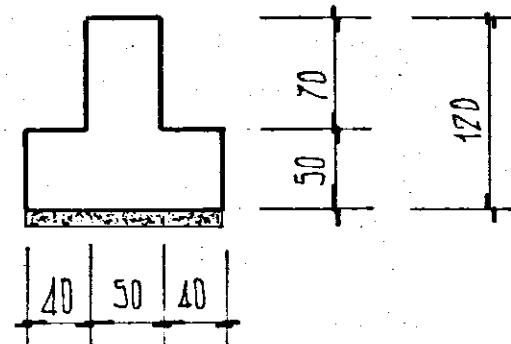
SEZ. D-D'
