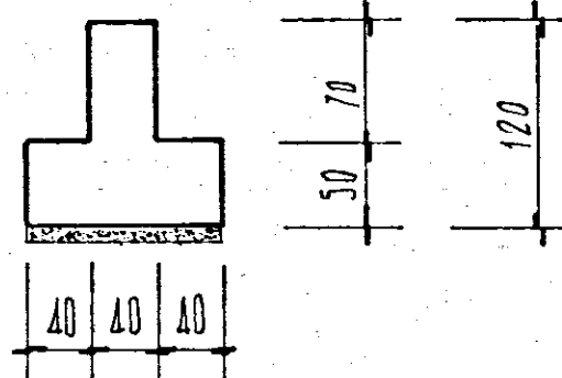
SEZ. C-C'
