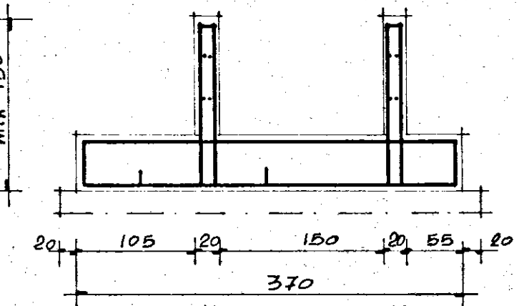
SEZ. B-10bis
