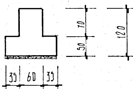
SEZ. B-B'
