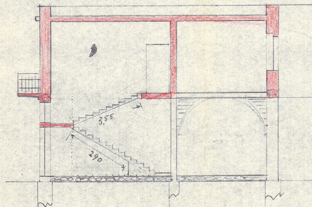
Sezione C-D
