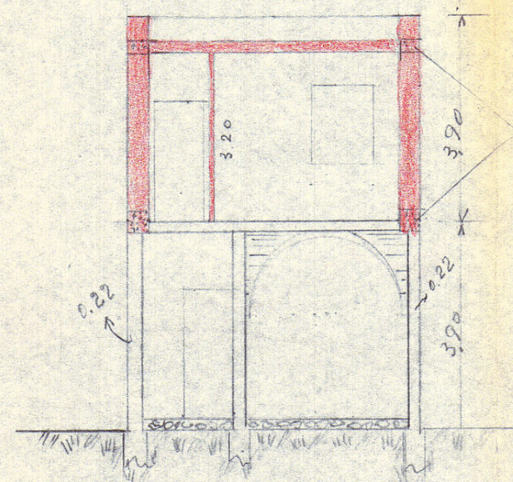
Sezione A-B
