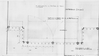
ESTERNO (0.30) SEZIONE ORIZZONTALE napp. 1:10
