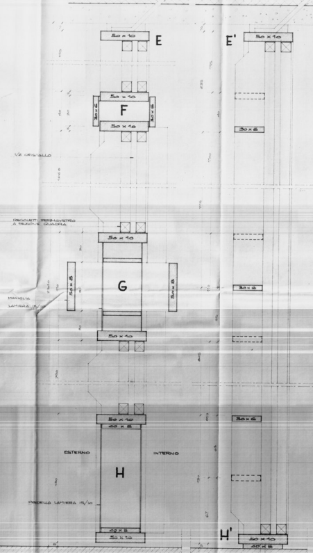
CANCELLO A VETRI NODI VERTICALI rapp. 1:1
